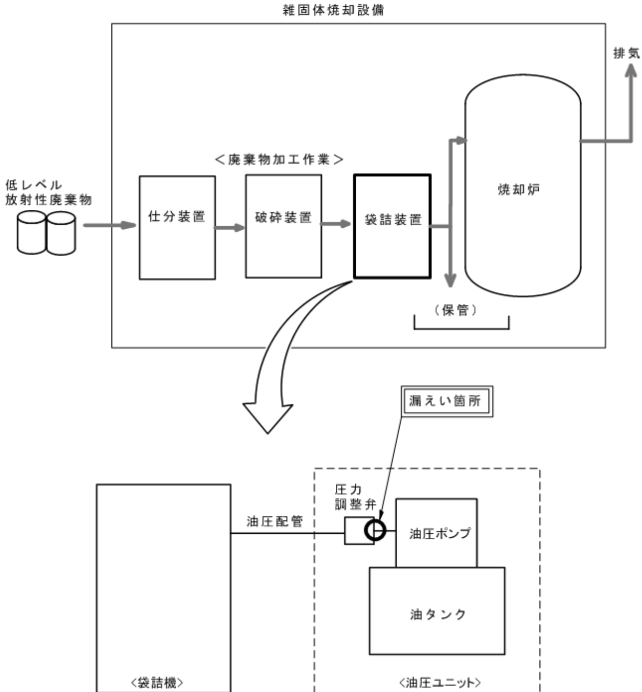
袋詰装置概略構成図
