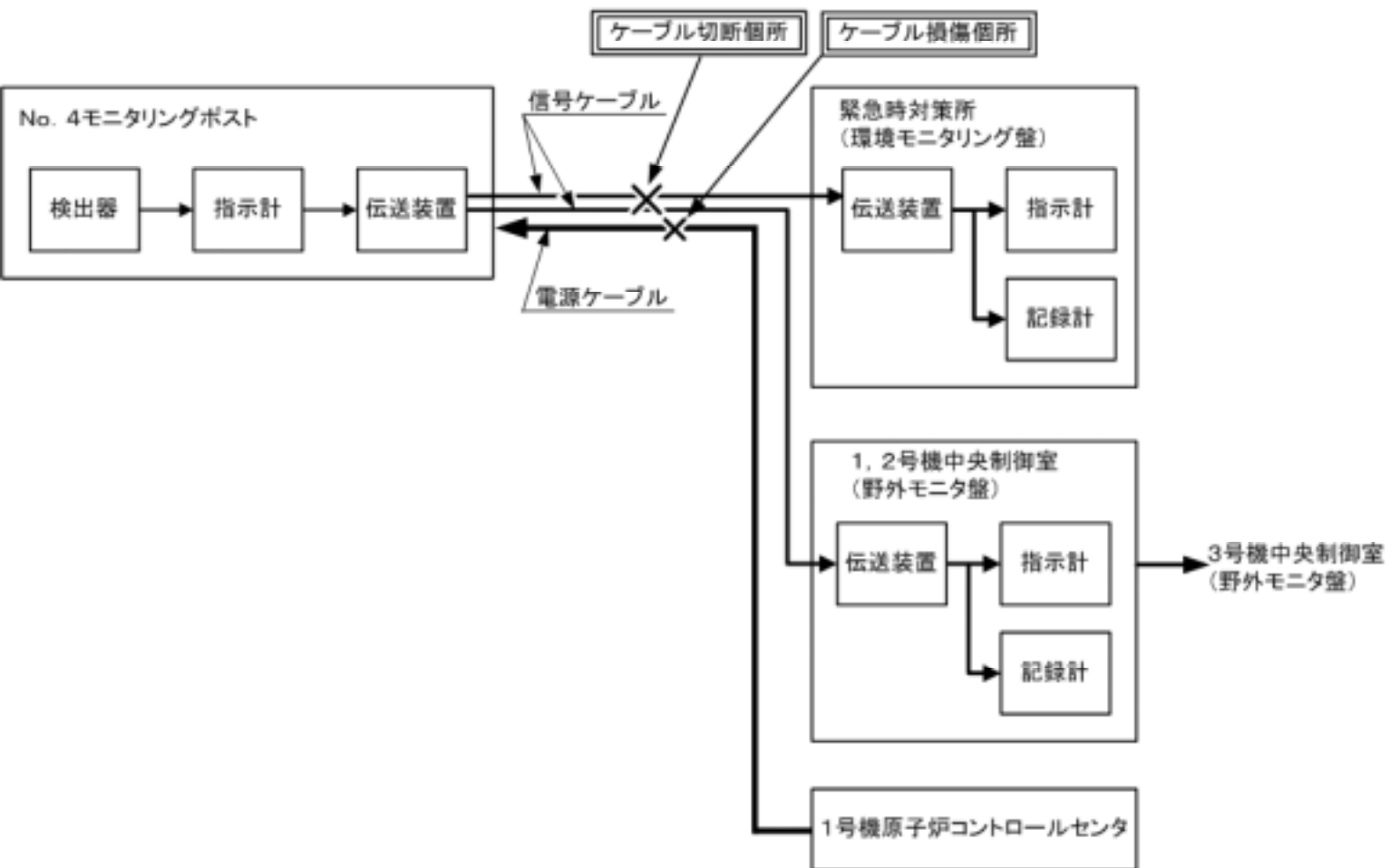
No. 4モニタリングポスト概略構成図
