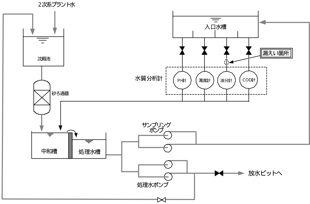
伊方3号機 総合排水処理装置サンプリングライン概略系統図
