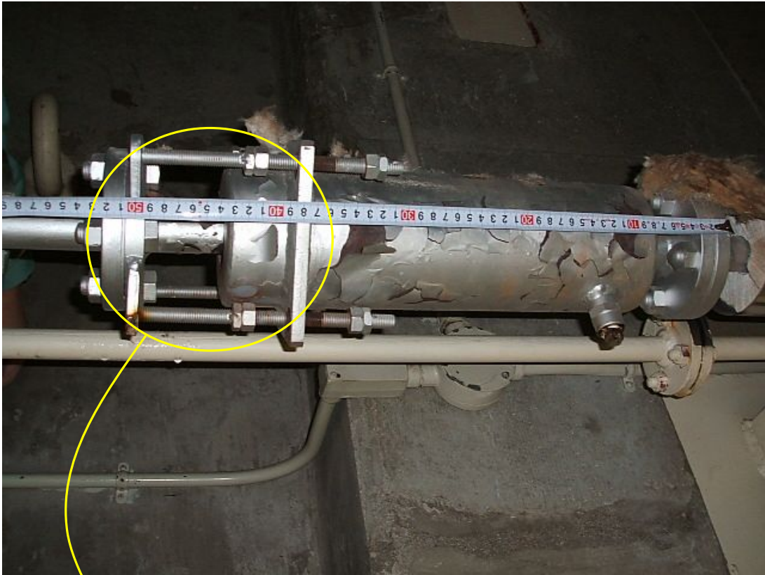
補助蒸気伸縮継手部全景
