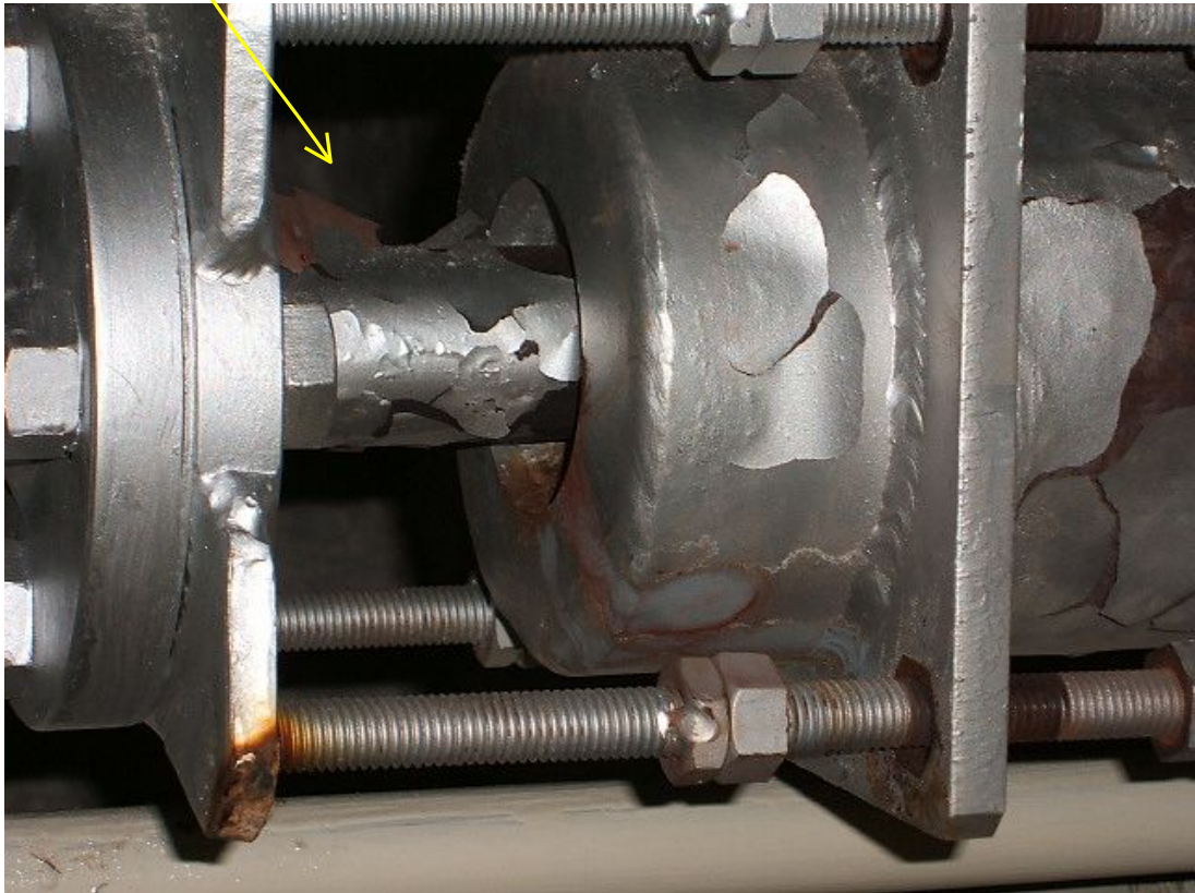
補助蒸気漏えい部
