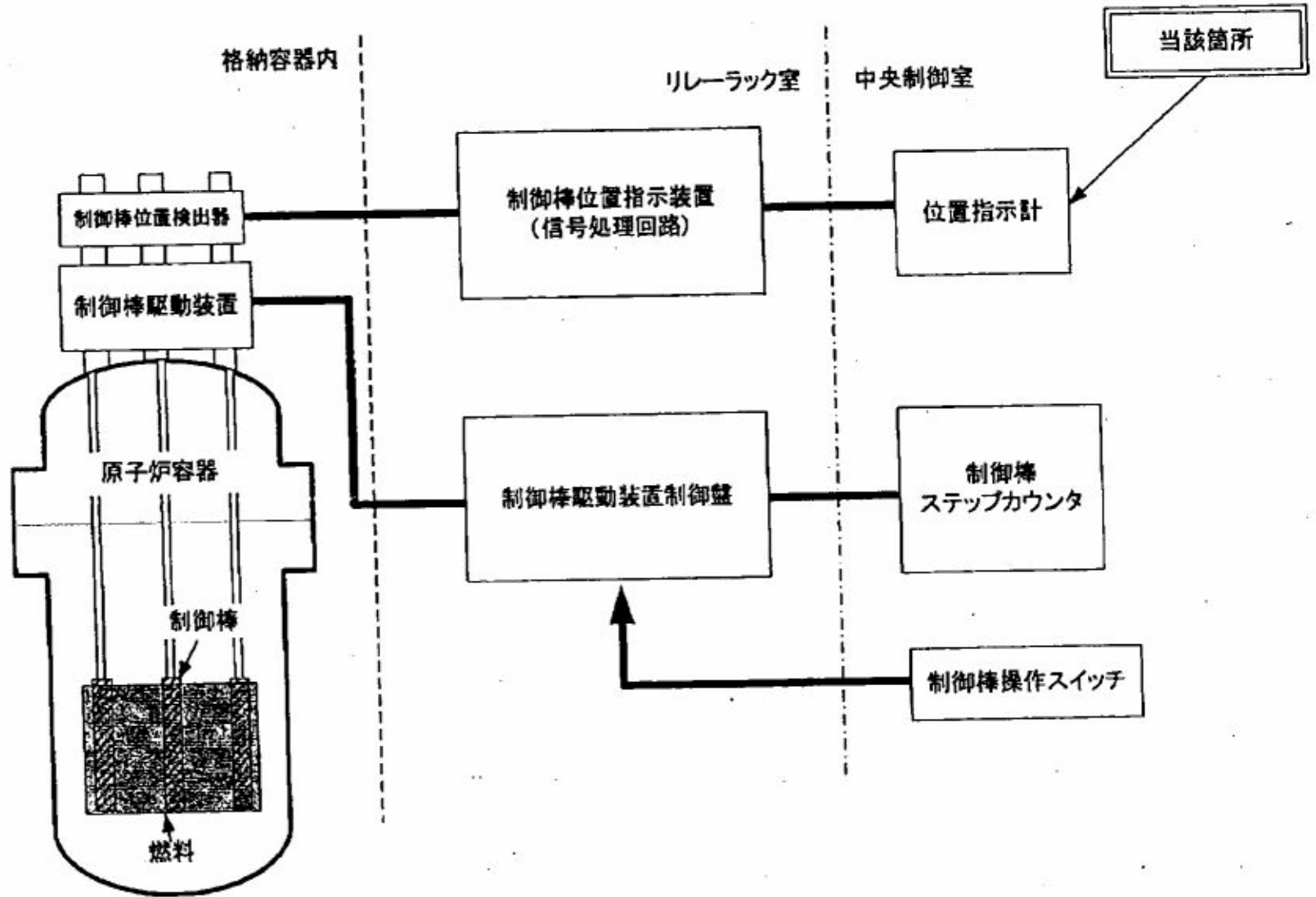
伊方発電所1号機制御棒位置指示装置概略系統図
