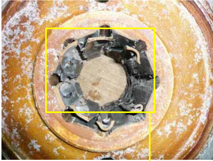
軸受摩耗状況
