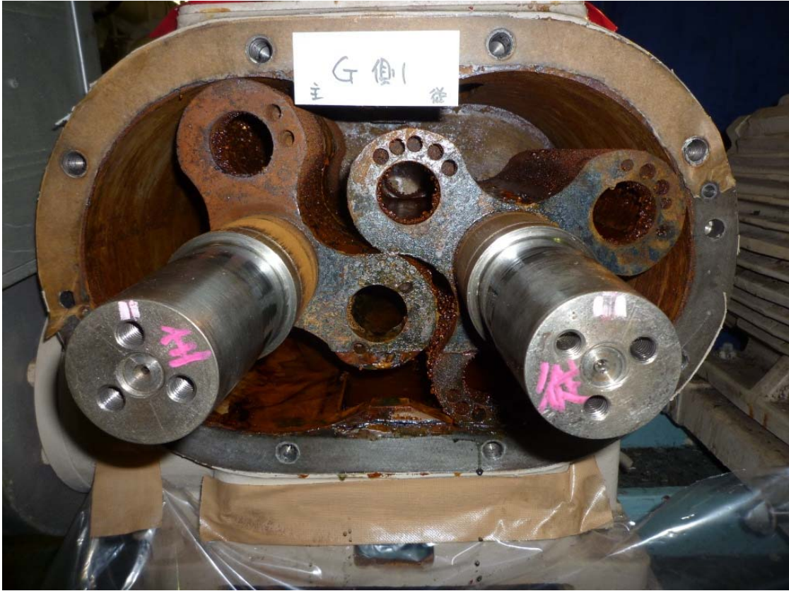
洗浄攪拌ブロワ（内部）の状況
