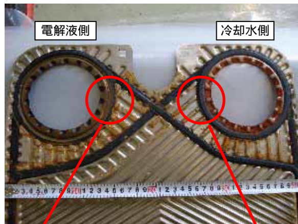
プレート(ガスケット)状況
