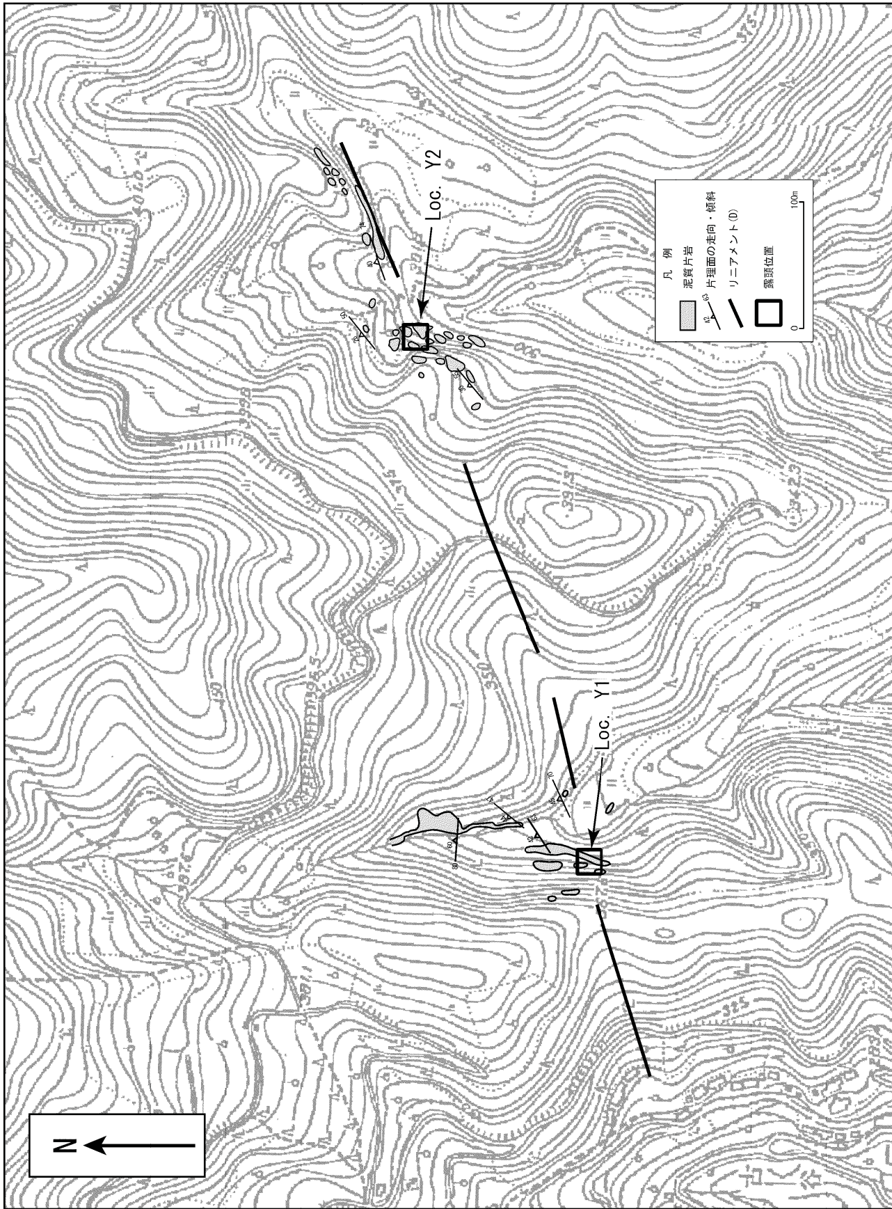
添付図-2.3：八幡浜リニアメント周辺のルートマップ(LOC. Y1, Y2) (国土地理院発行5千分の1国土基本図を使用)
