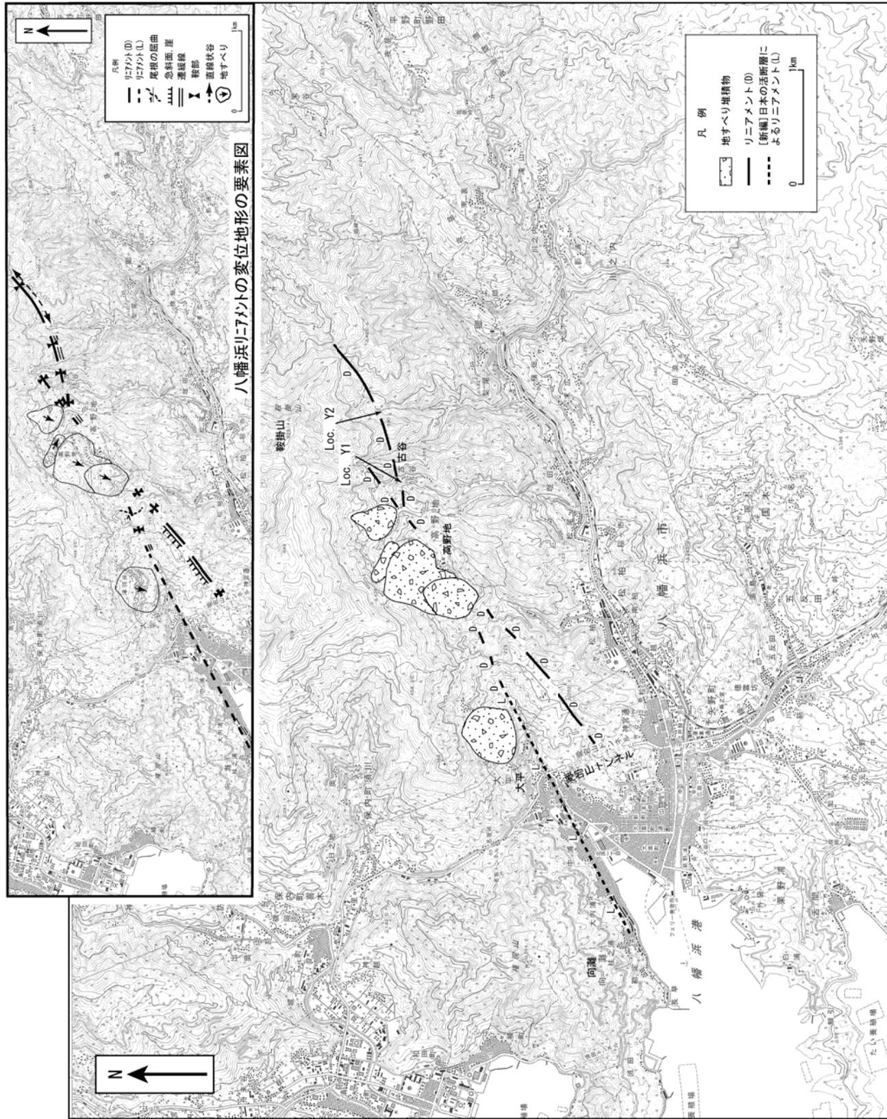
添付図-2.1：八幡浜リニアメント周辺の変位地形・リニアメント分布図(国土地理院発行数値地図25000(地図画像)を使用)
