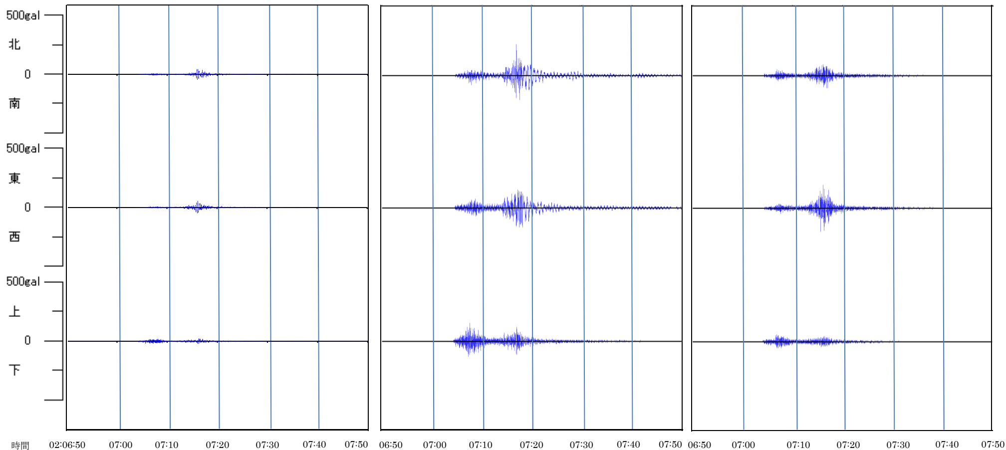
伊方発電所1号機原子炉補助建家基礎上端
