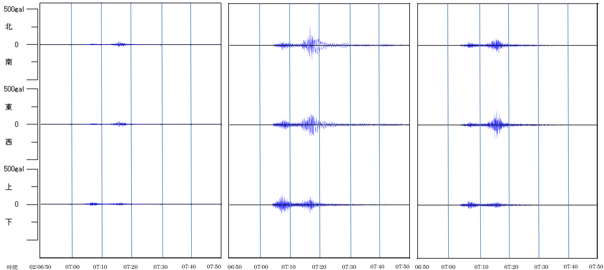
伊方発電所3号機原子炉補助建屋基座上端
