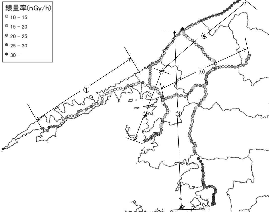
図1-1 3"φ×3" NaI (Tl) シンチレーション検出器 (エネルギー補償方式) による測定結果 (地図上データ表示) (平成25年6月測定結果)
