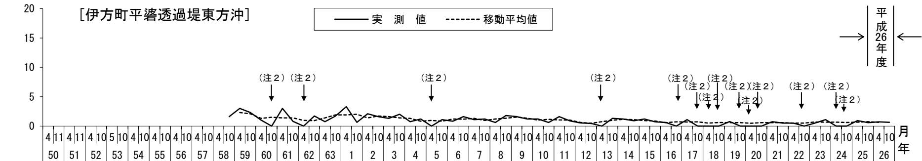
図37 海底土中のセシウム-137濃度の推移 (四国電力(株)測定分)
