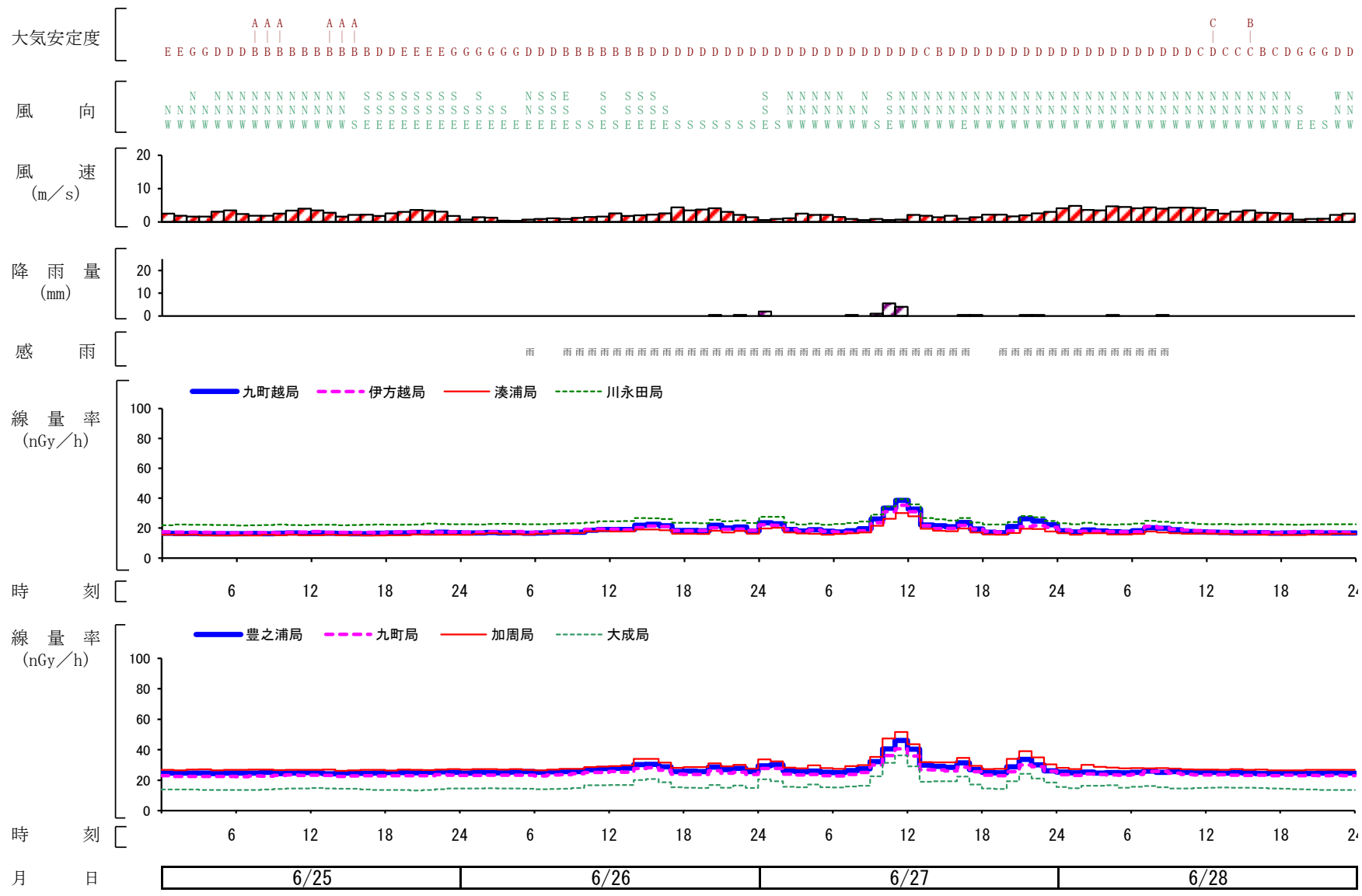
図8 降雨に対応して発生している線量率の変化例 平成26年06月25日～平成26年06月28日
