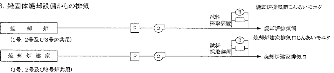
第 8.1 図 解体工事準備期間の放射性気体廃棄物の処理フロー
