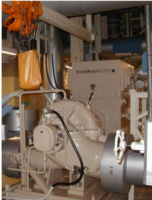
補機冷却水ポンプ全景
