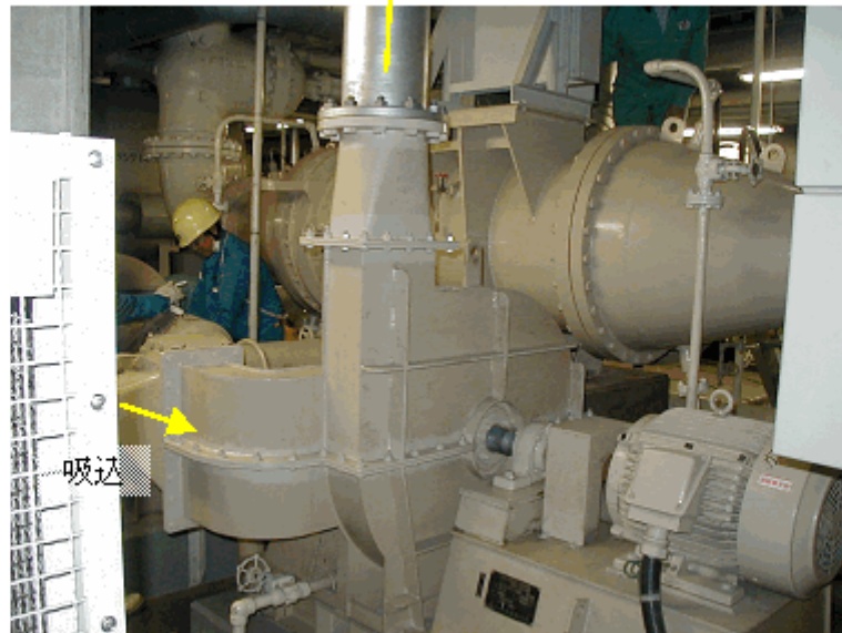
グラウンド蒸気排風機全景
