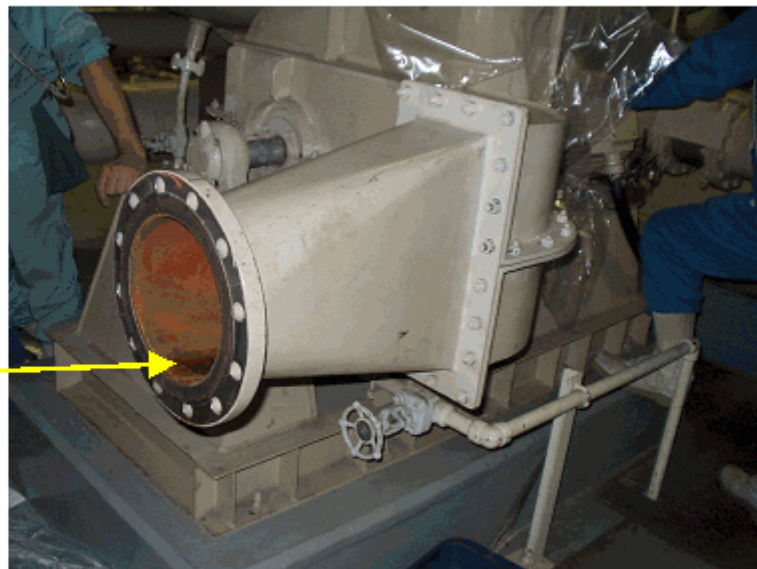
グラウンド蒸気排風機 吸込部
