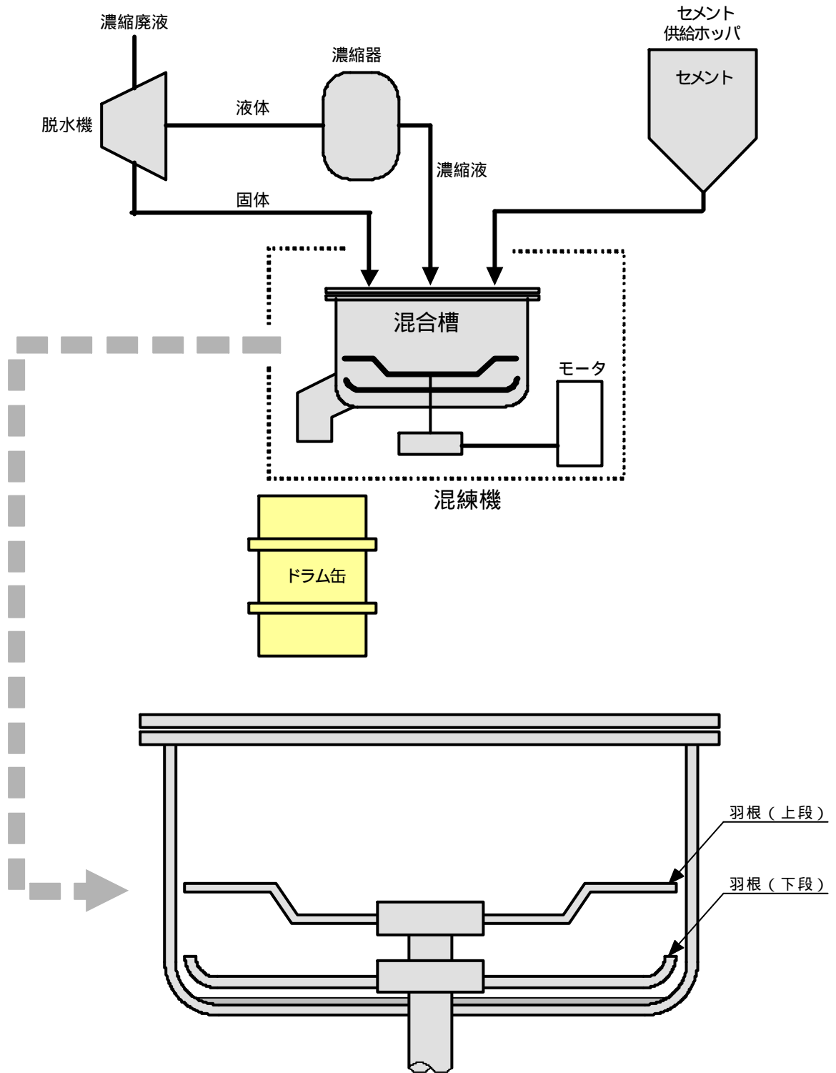
混合槽の概略構造図
