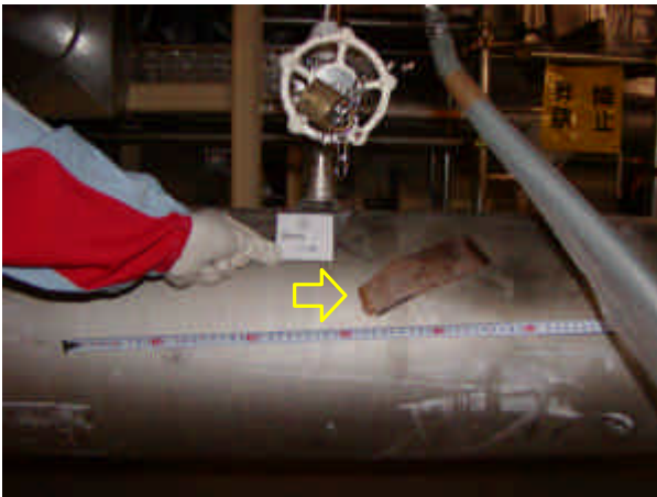
余熱除去系統配管テープ状附着物確認部 (PT 調査中)
