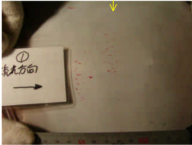
液体浸透探傷検査(PT)指示部
