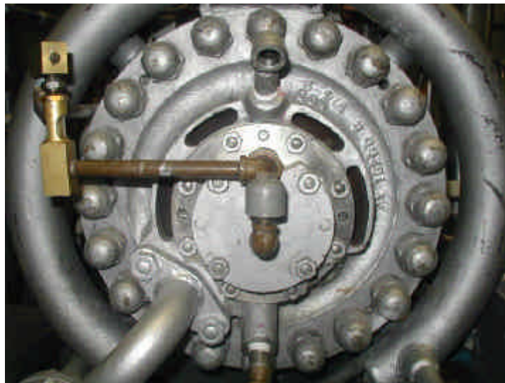
ポンプ軸端側軸封部
