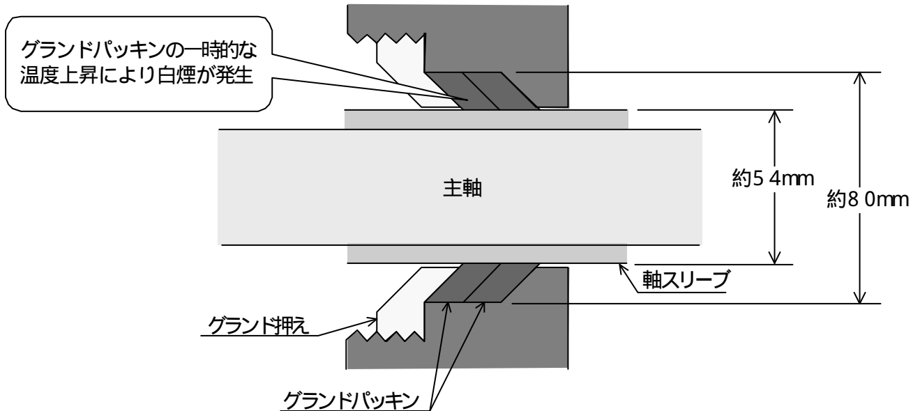
軸封部拡大図
