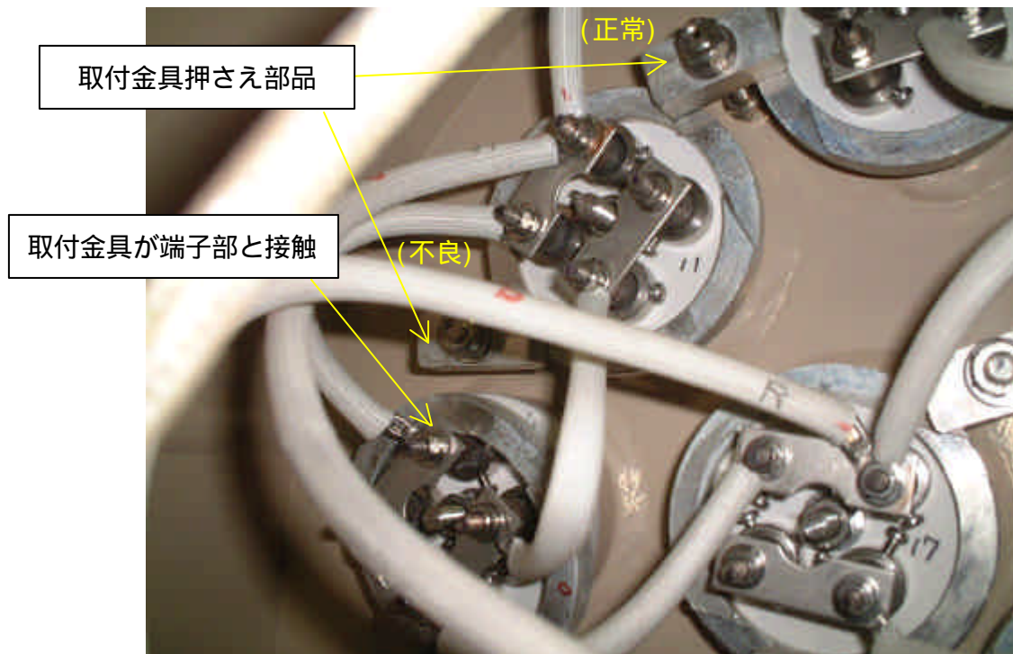
非常用ディーゼル発電機清水加熱器 ヒーター端子部
