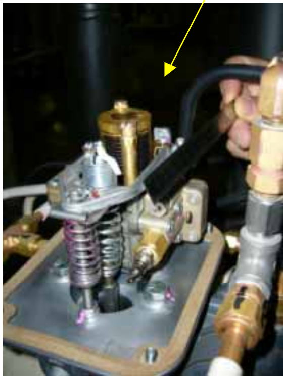
脱気器加熱蒸気圧力制御弁の制御機構部
