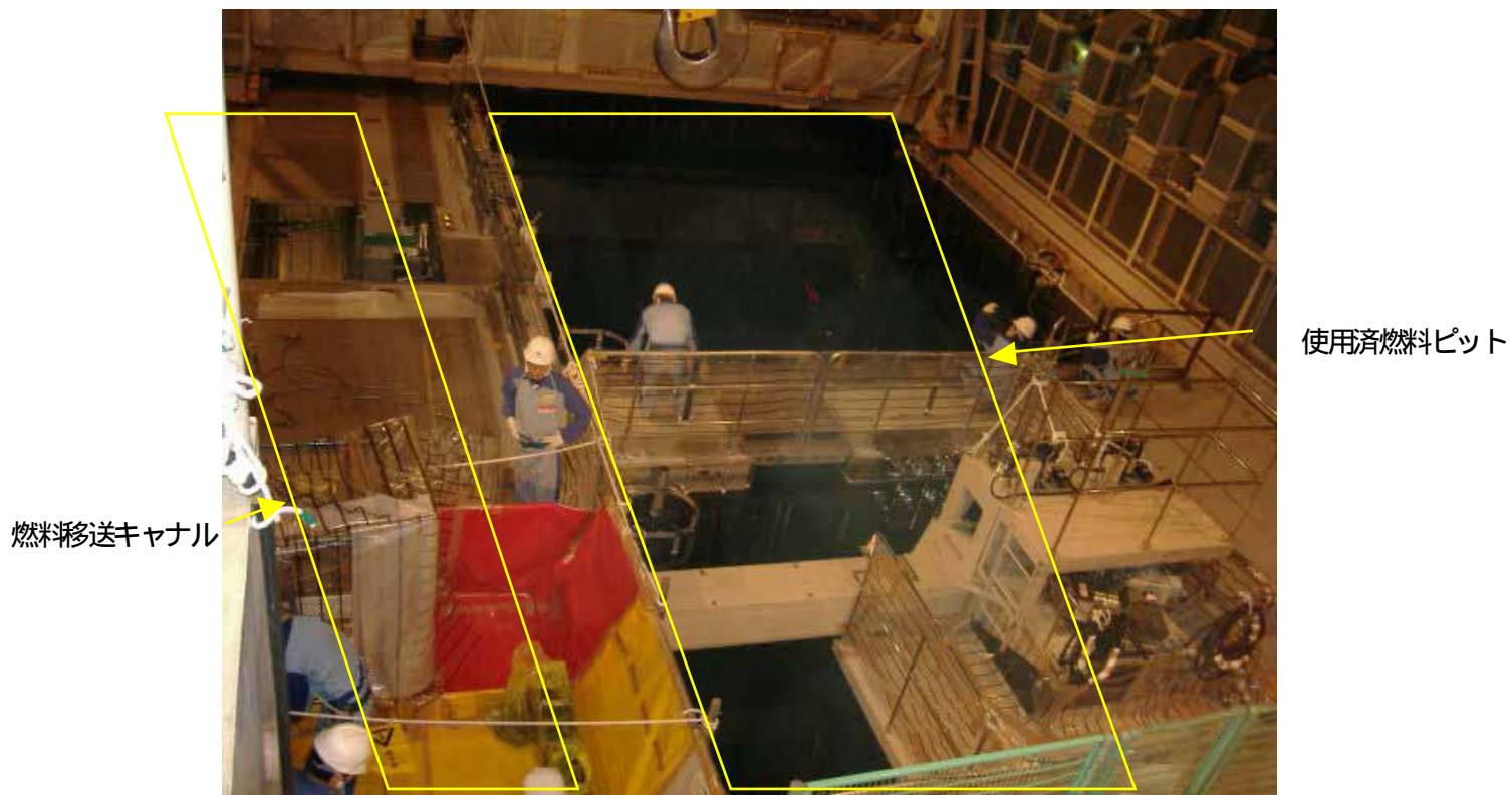
使用済燃料ピット及び燃料移送チャンネル
