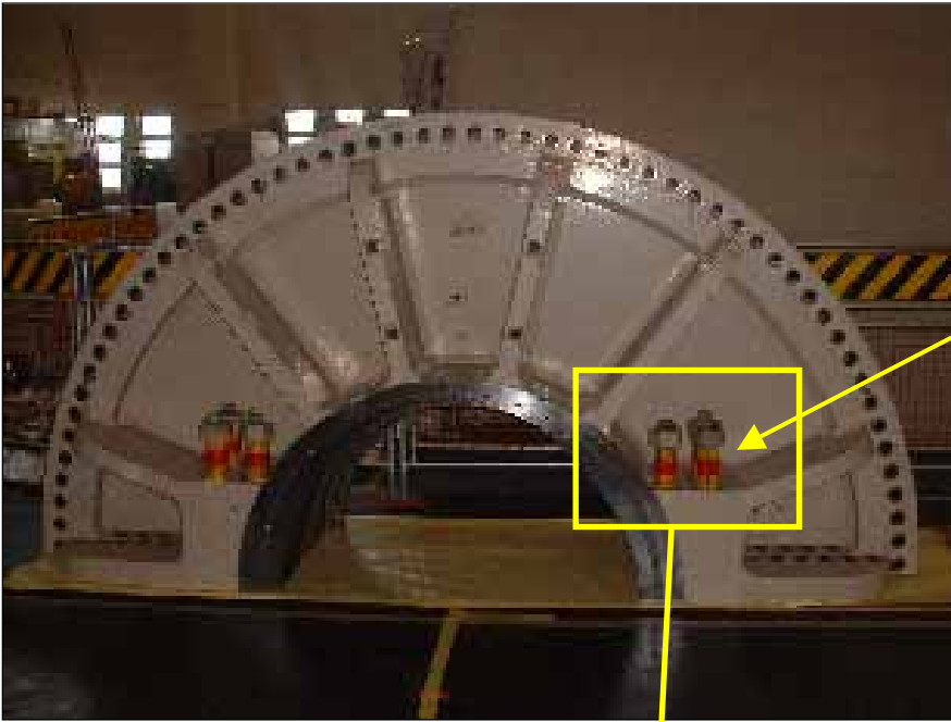
タービン発電機上部カバー写真
