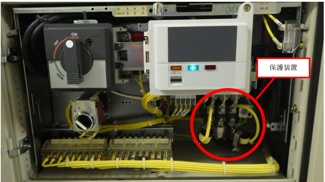
電源ユニット (グラント蒸気復水器排気ファン)
