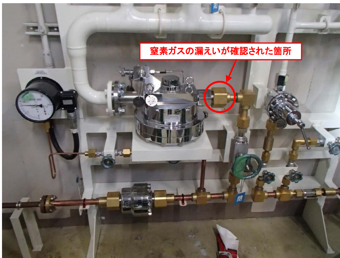
発電機用窒素ガス封入装置
