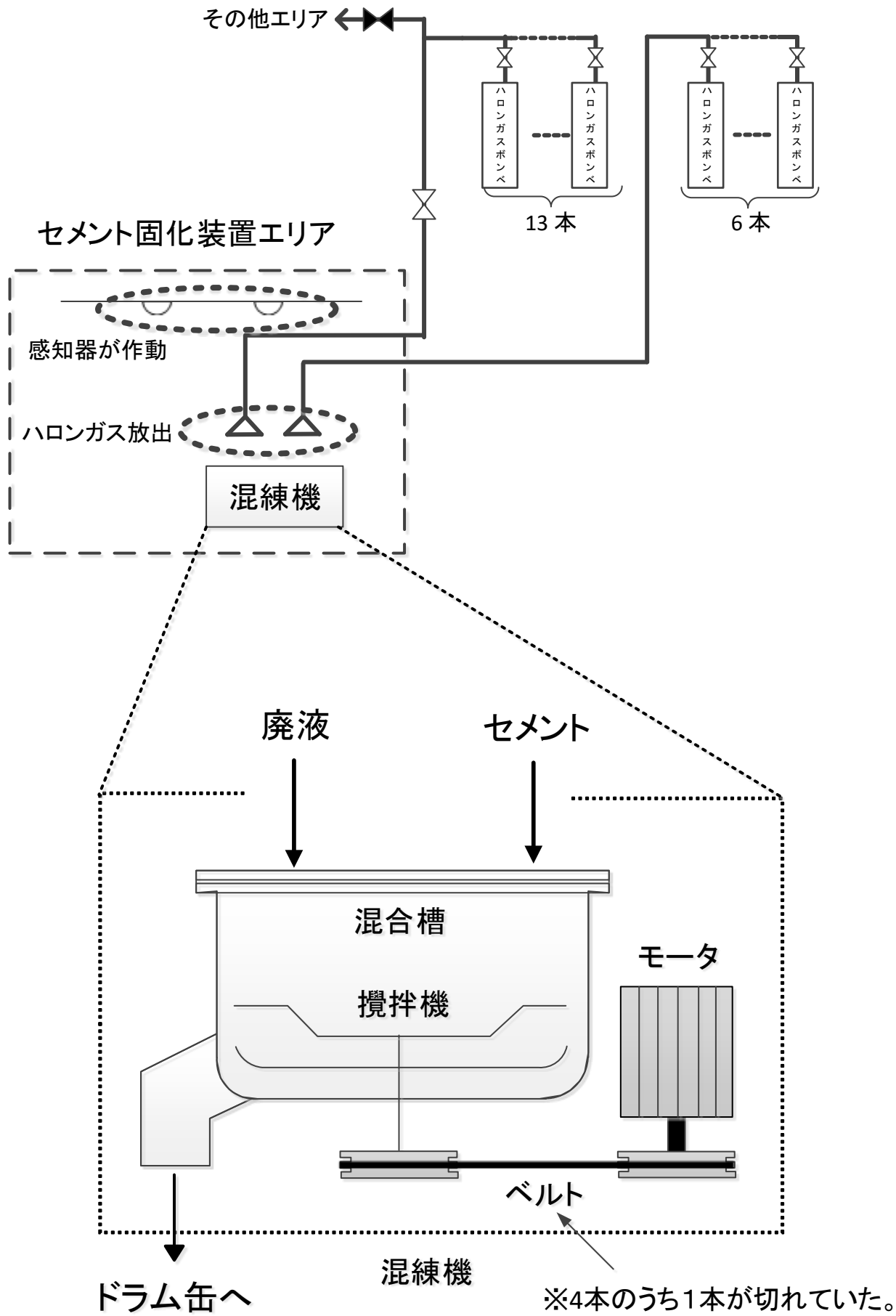
混練機概略図
