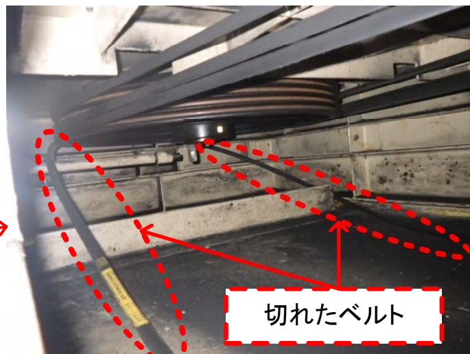
モータと攪拌機を連結しているベルトの状態
