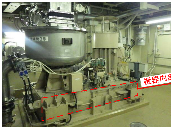
セメント固化装置混練機(全体)
