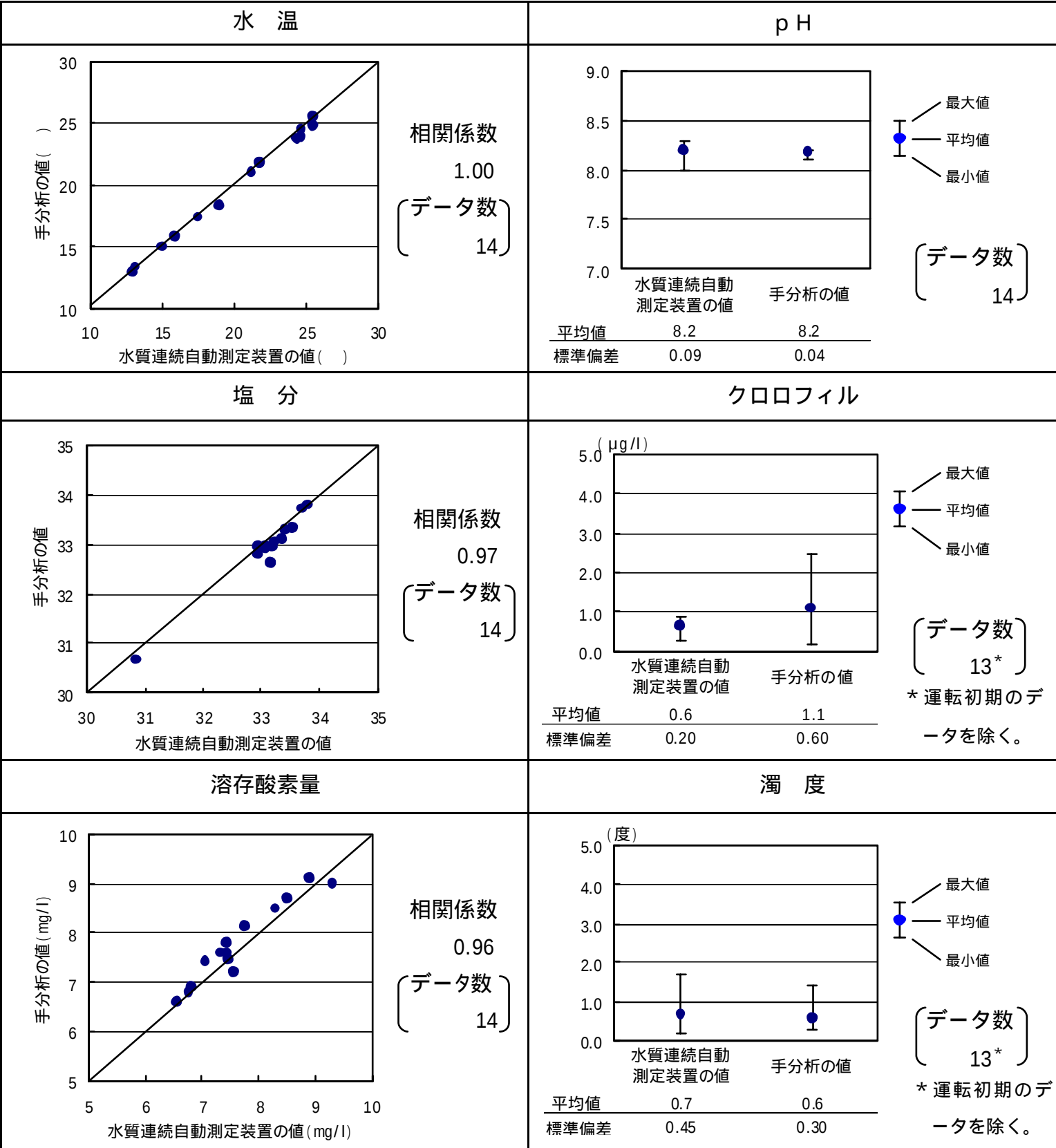
図1 水質連続自動測定装置と手分析の値の比較
