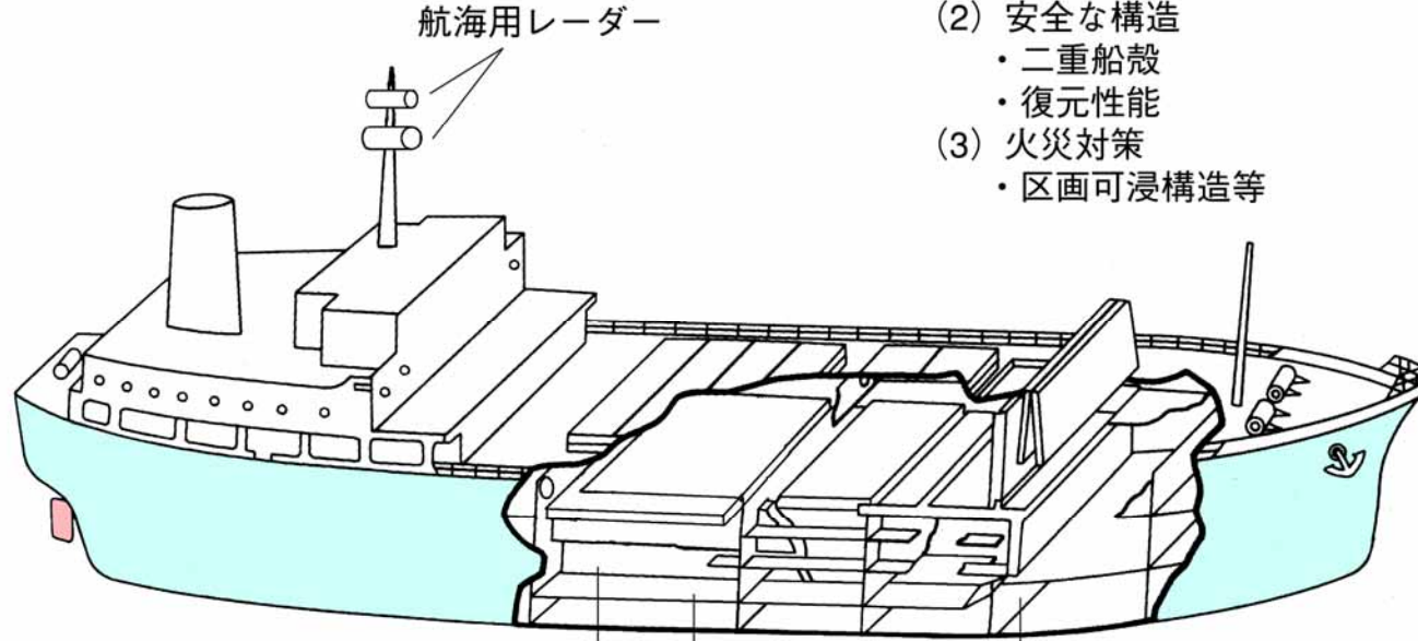
船体断面図
