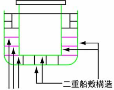
船体断面図
