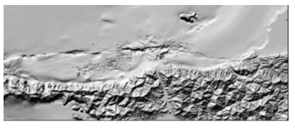
海底地形
