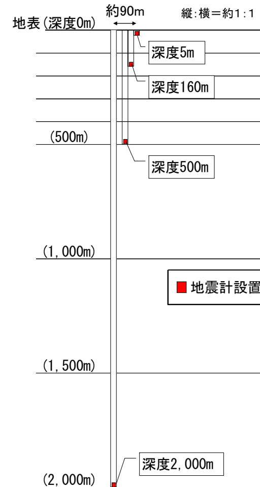
地震計設置断面図
