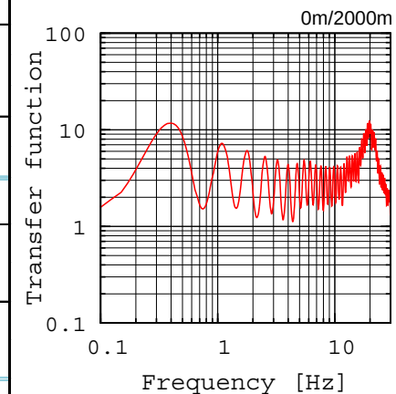
鉛直アレイモデルによる 理論伝達関数
