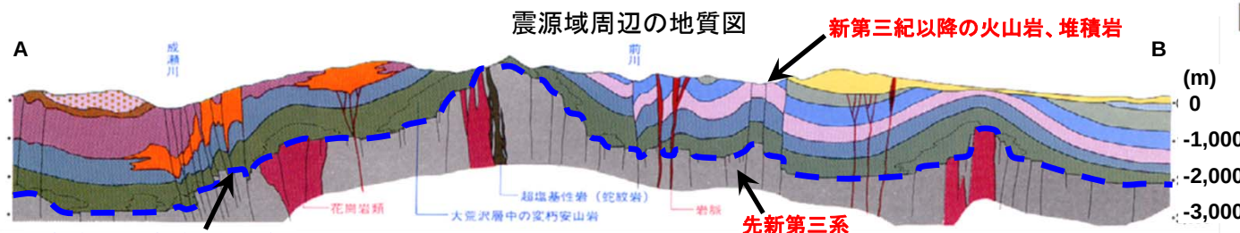
地質断面図 (南北幅数kmの範囲を投影)
