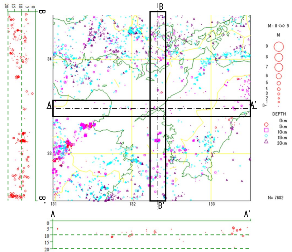
気象庁一元化震源
