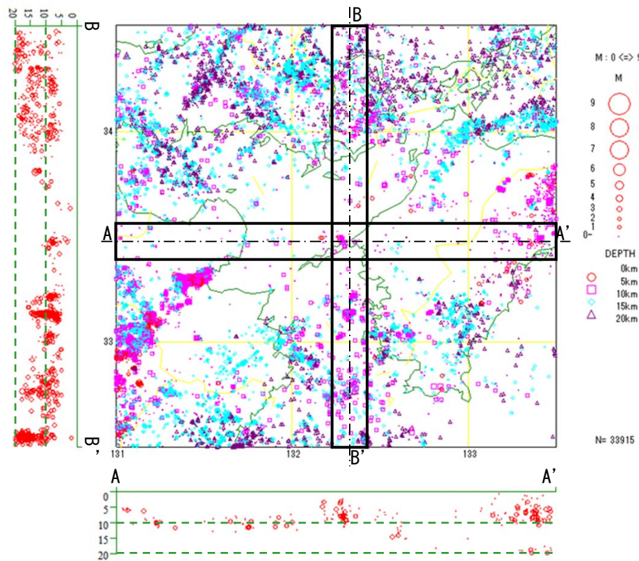
気象庁一元化震源
