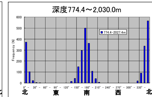
＜H23.3.11地震後のブレイクアウト方位＞
