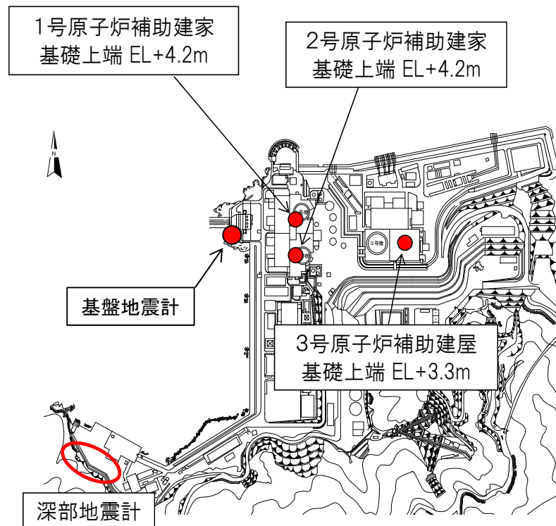
地震計設置位置図(配置図)
