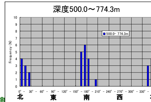
＜H23.3.11地震前のブレイクアウト方位＞
