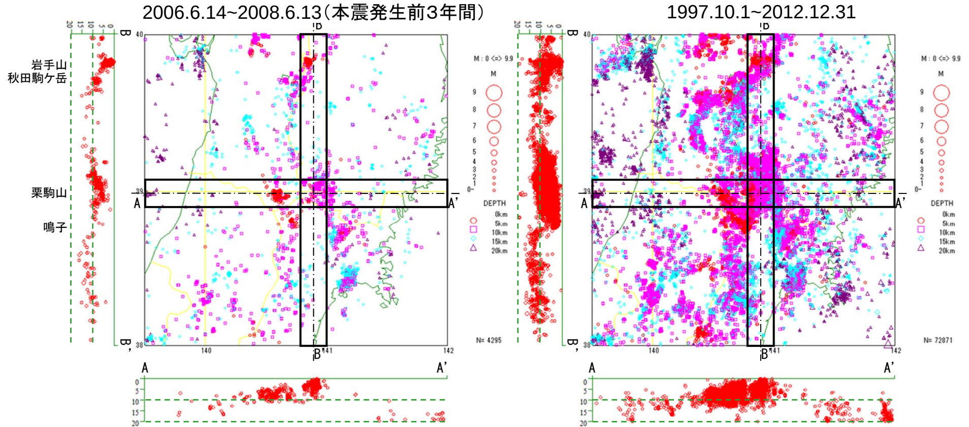
気象庁一元化震源
