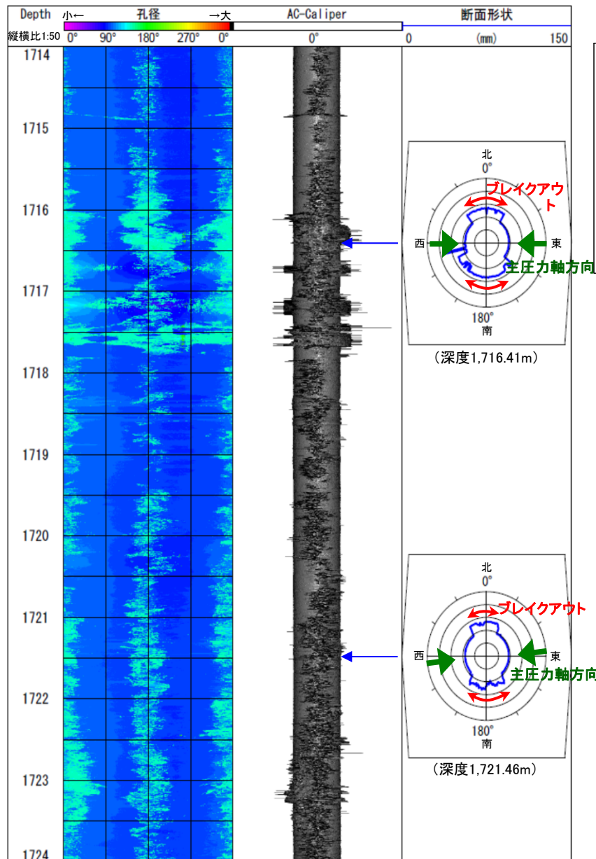
＜H23.3.11地震前のブレイクアウト方位＞
