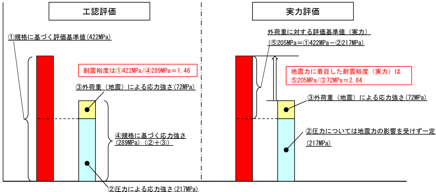
図1 実力評価方法のイメージ図(原子炉容器管台の例)
