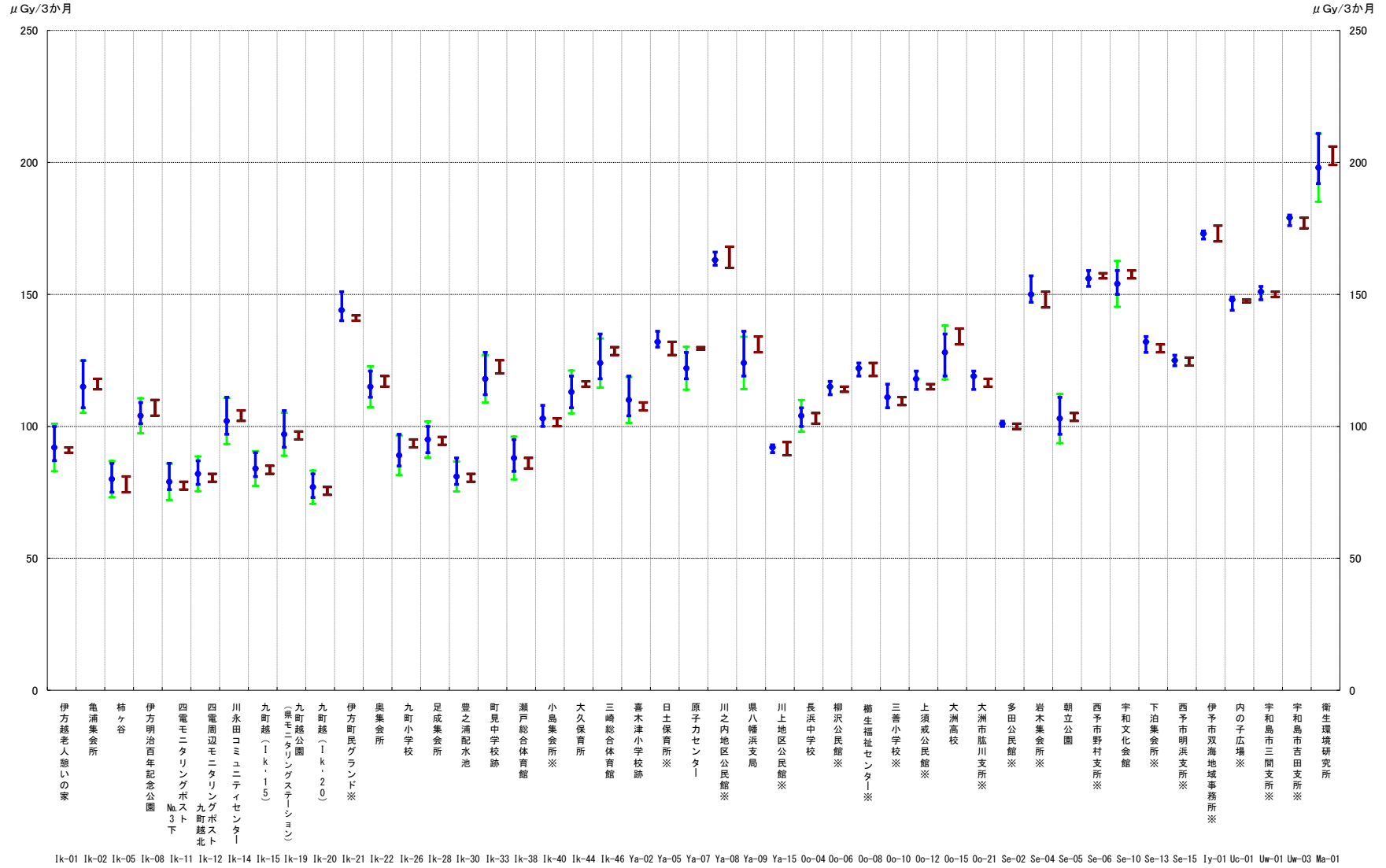
図30 積算線量測定結果の過去における測定値との比較図（愛媛県測定分）
