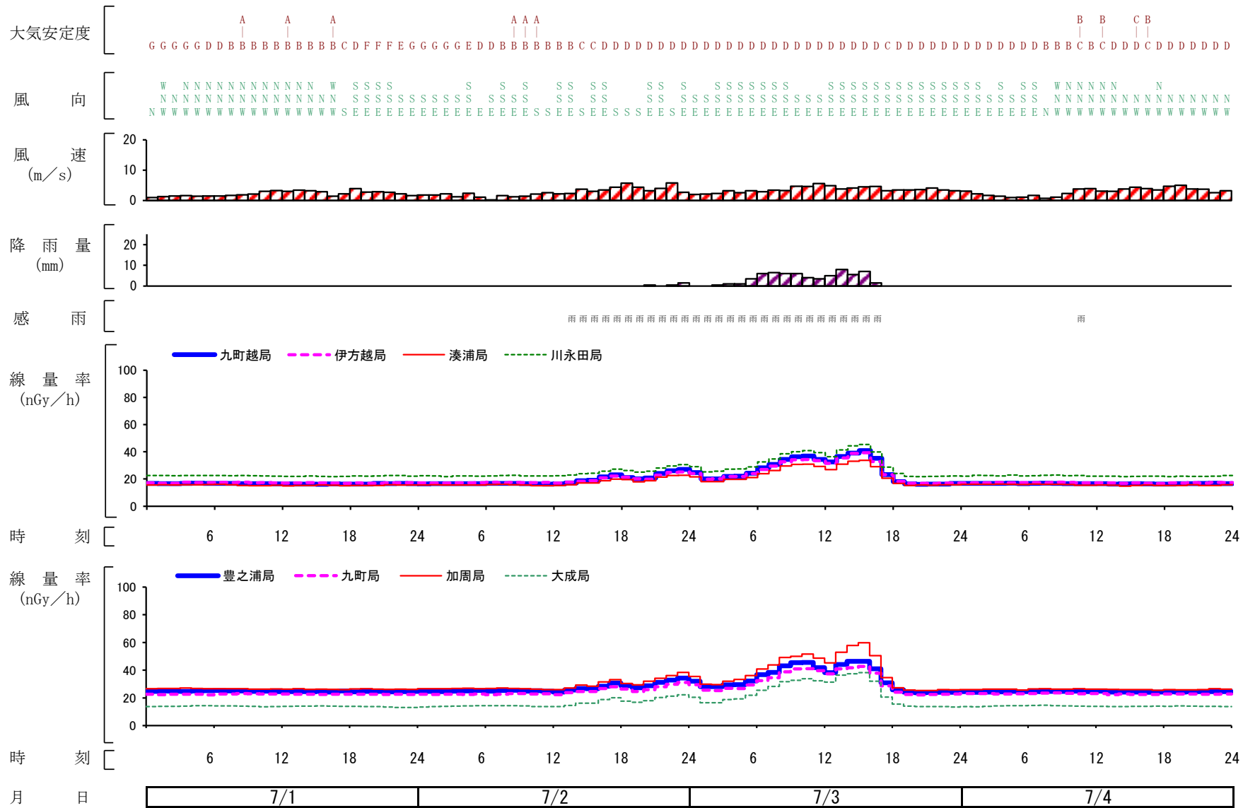
図9 降雨に対応して発生している線量率の変化例 平成26年07月01日～平成26年07月04日
