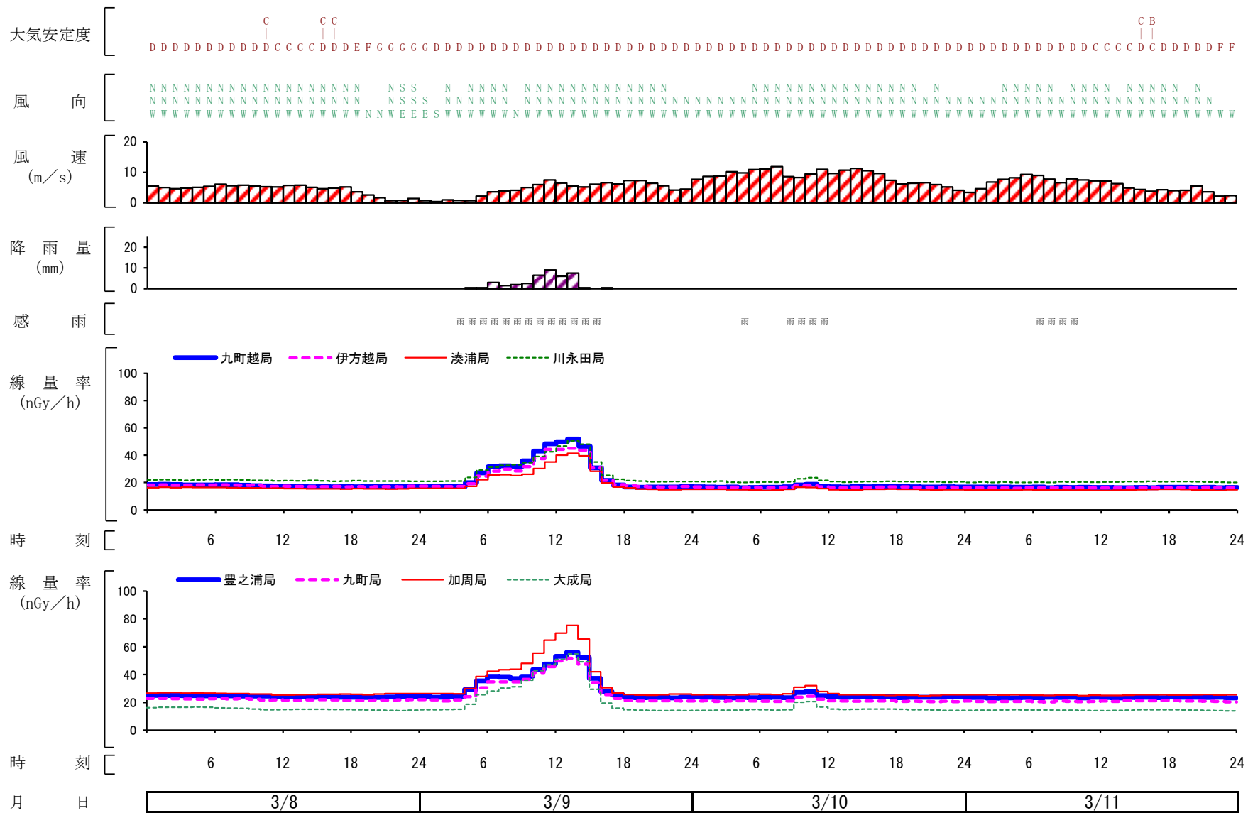
図11 降雨に対応して発生している線量率の変化例 平成27年03月08日～平成27年03月11日
