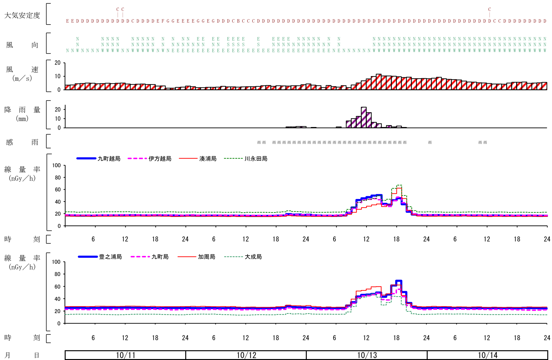
図10 降雨に対応して発生している線量率の変化例 平成26年10月11日～平成26年10月14日
