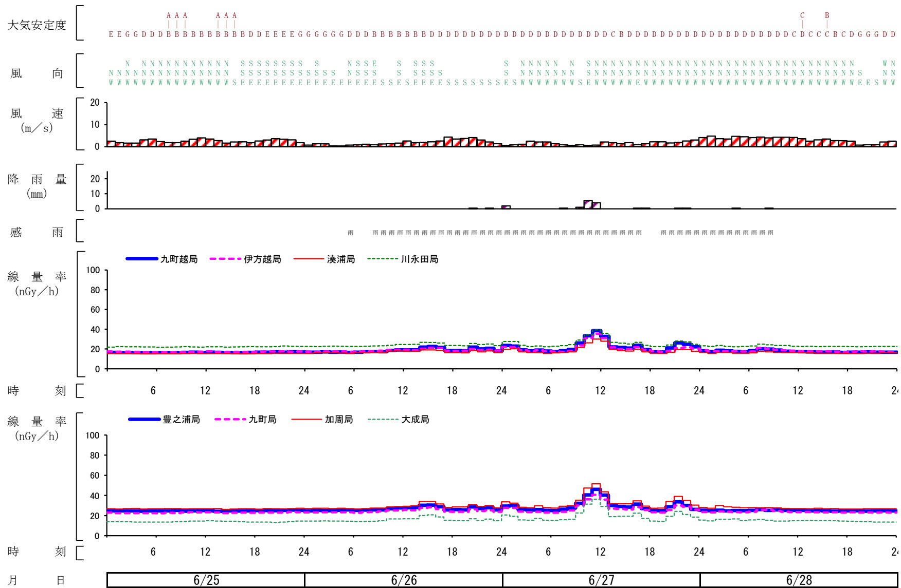
図8 降雨に対応して発生している線量率の変化例 平成26年06月25日～平成26年06月28日
