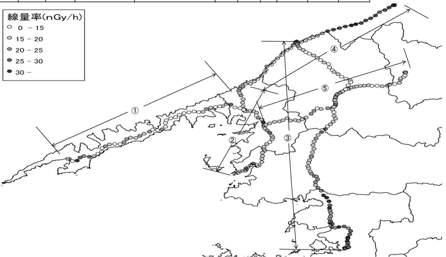
図1-1 3"φ×3" NaI (Tℓ) シンチレーション検出器 (エネルギー補償方式) による測定結果(地図上データ表示) (平成26年6月測定結果)
