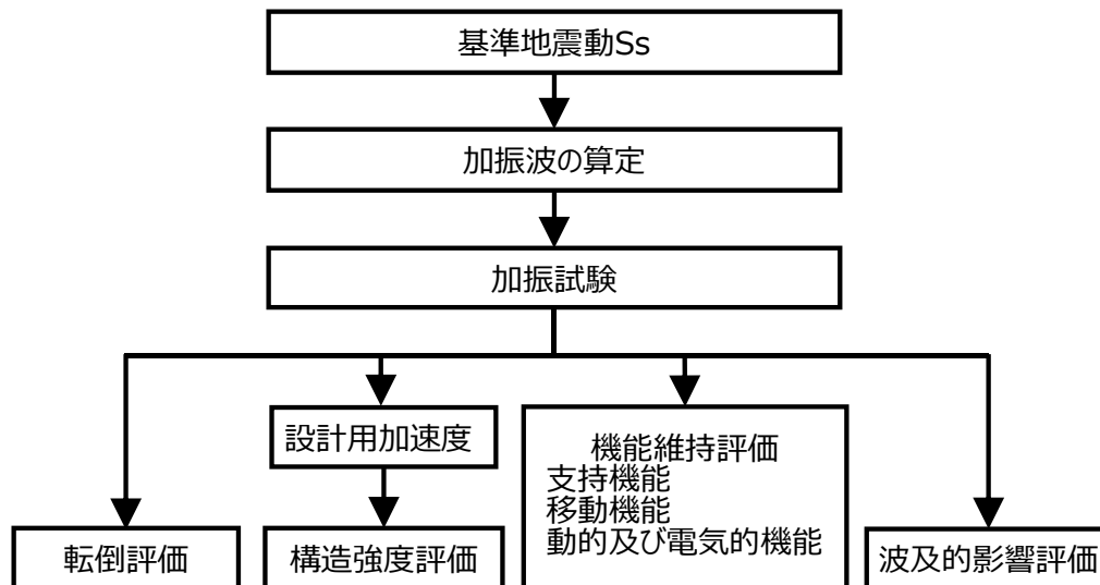
耐震評価フロー
