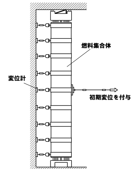
自由振動試験概要図 (例：A型燃料集合体)
