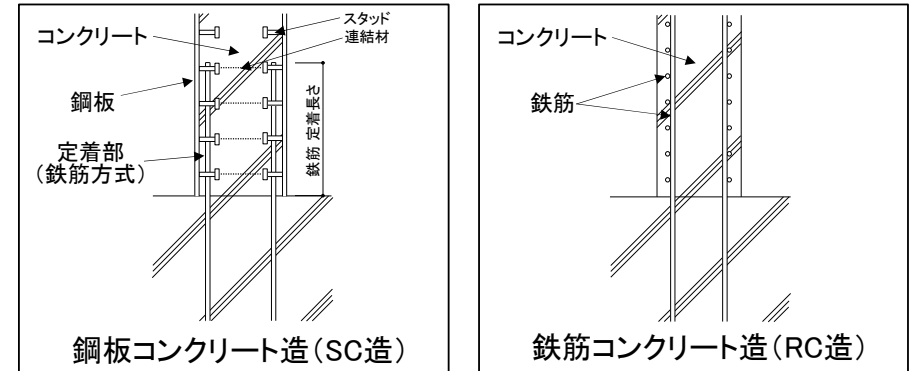
構造概念図
