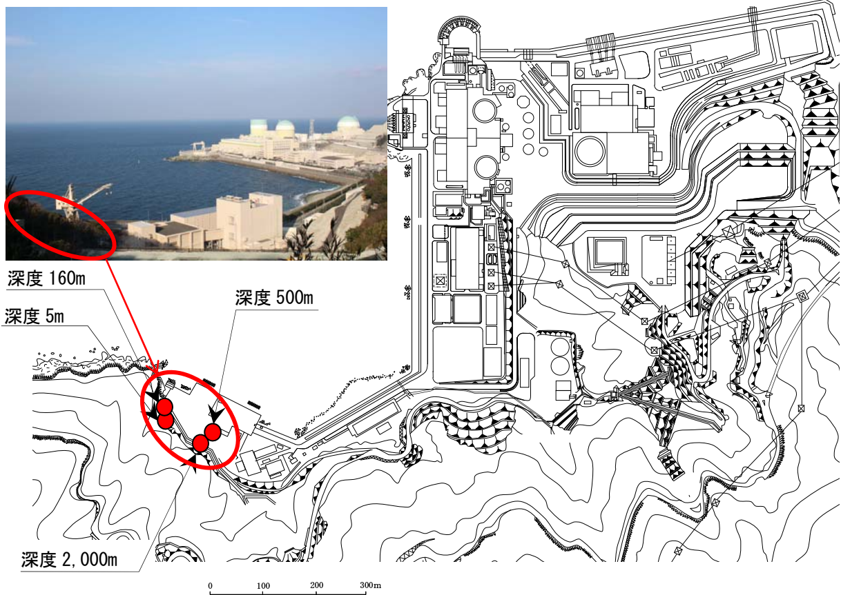
図 深部地震計の設置場所
