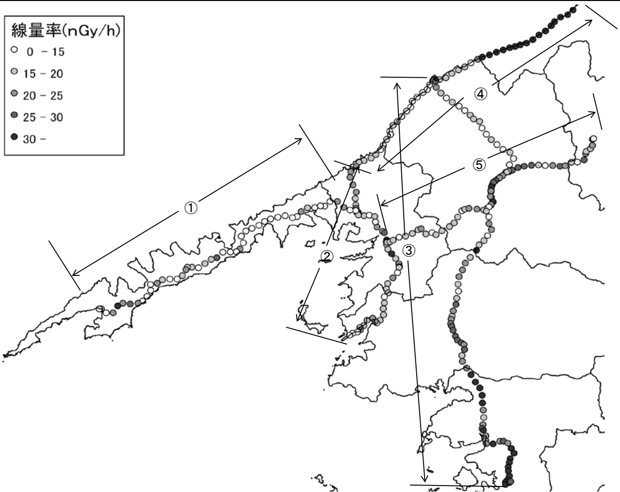
図2-3 球形3"φNaI (Tl) シンチレーション検出器による測定結果(地図上データ表示) (平成30年9月測定結果)
