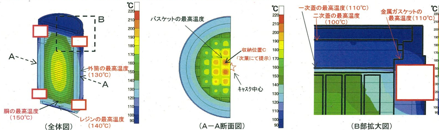
【温度分布図】<タイプ1> 1,2号炉ウラン燃料(14×14型燃料)用(発熱量: 16.9kW)
