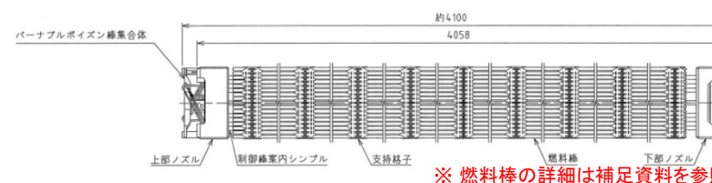
【使用済燃料の構造図(17×17型燃料の例)】
