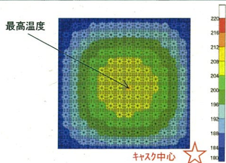
【温度分布図】 使用済燃料集合体断面(収納位置C) <タイプ1> 1,2号炉ウラン燃料(14×14型燃料)用(発熱量:16.9kW)
