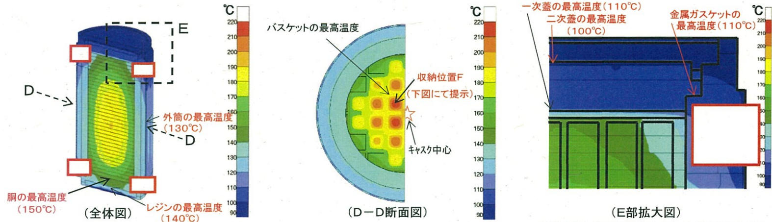
【温度分布図】<タイプ2> 3号炉ウラン燃料(17×17型燃料)用(発熱量:18.1kW)
