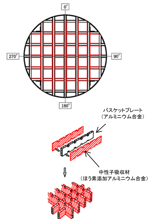
【バスケット構造図(1, 2号炉燃料用の例)】
