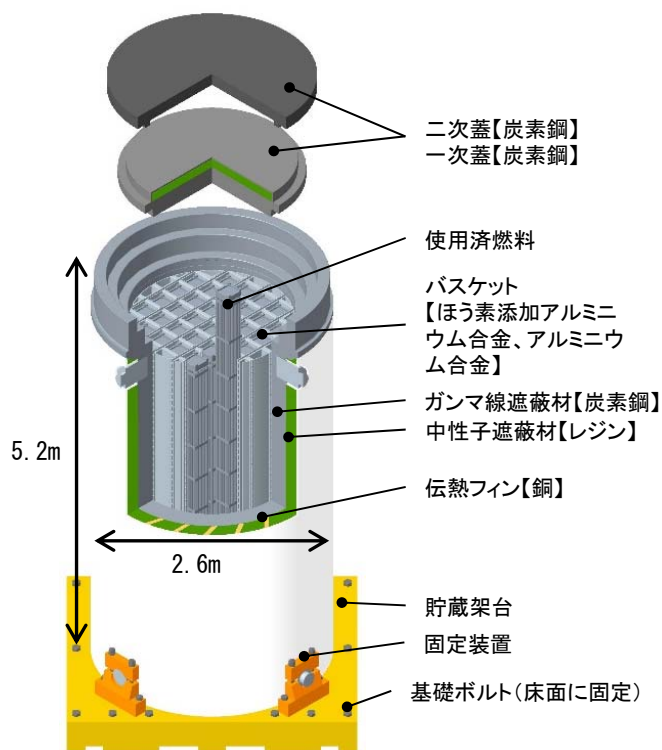
【乾式キャスクの構造図】
