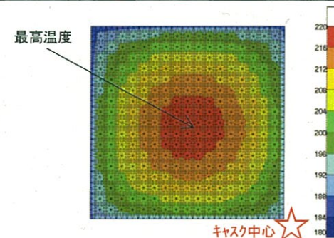
【温度分布図】 使用済燃料集合体断面(収納位置F) <タイプ2> 3号炉ウラン燃料(17×17型燃料)用(発熱量:18.1kW)
