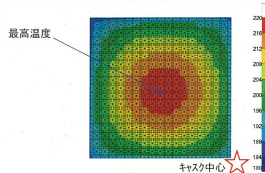
【温度分布図】 使用済燃料集合体断面(収納位置F) <タイプ2> 3号炉ウラン燃料(17×17型燃料)用(発熱量: 18.1kW)
