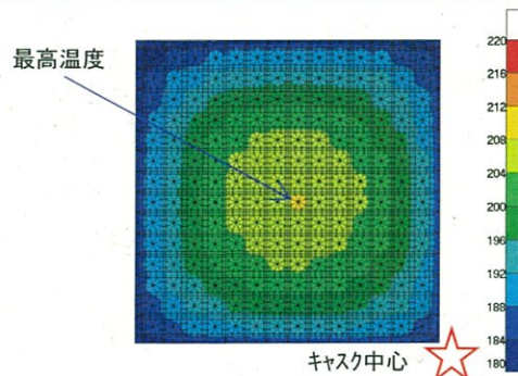
【温度分布図】 使用済燃料集合体断面(収納位置C) <タイプ1> 1,2号炉ウラン燃料(14×14型燃料)用(発熱量: 16.9kW)
