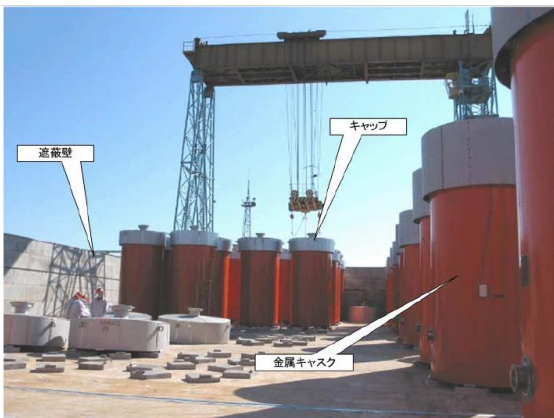
遮蔽壁方式
