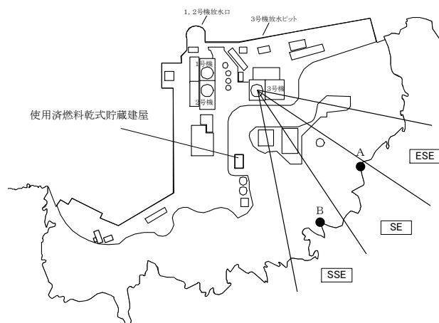
図 14 敷地境界外における年間線量解析結果
