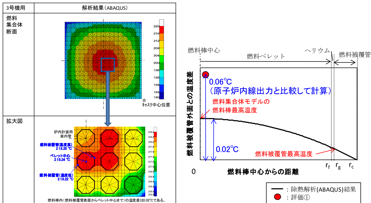
図 18 除熱解析における詳細結果
