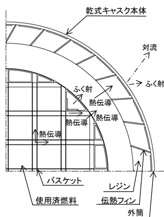
図16 乾式キャスクの除熱構造及び伝熱経路
