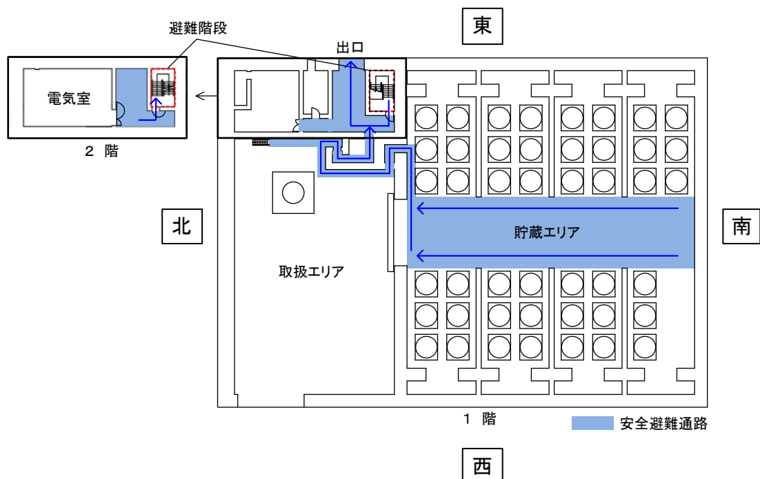
図 8 乾式貯蔵建屋の安全避難通路等
