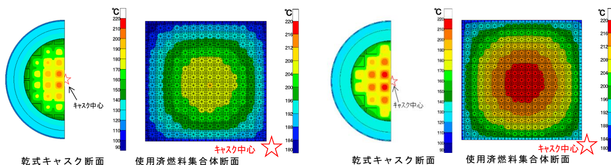
【温度分布図】
