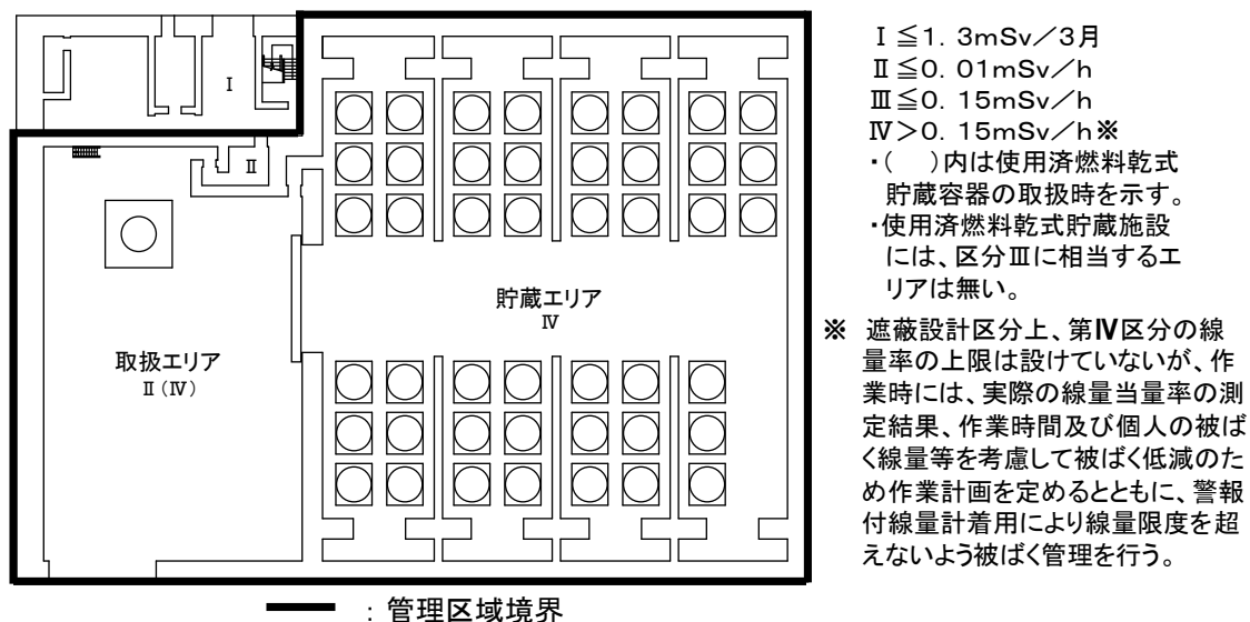
図 15 乾式貯蔵施設の管理区域
