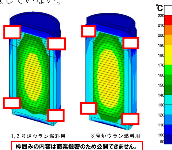
図17 除熱解析の3次元評価結果
