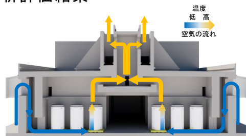
図10 乾式貯蔵建屋の除熱機能
