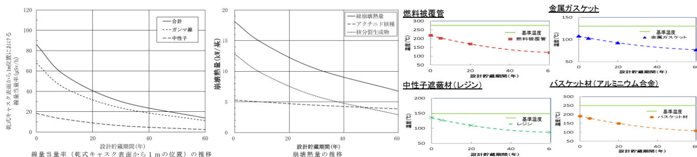
図 19 3号機ウラン燃料用乾式キャスクにおける線量当量率等の経年変化
