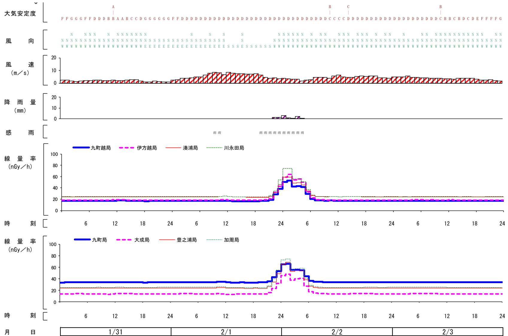
図 12 降雨に対応して発生している線量率（1時間平均値）の変化例（令和3年1月31日～令和3年2月3日）
