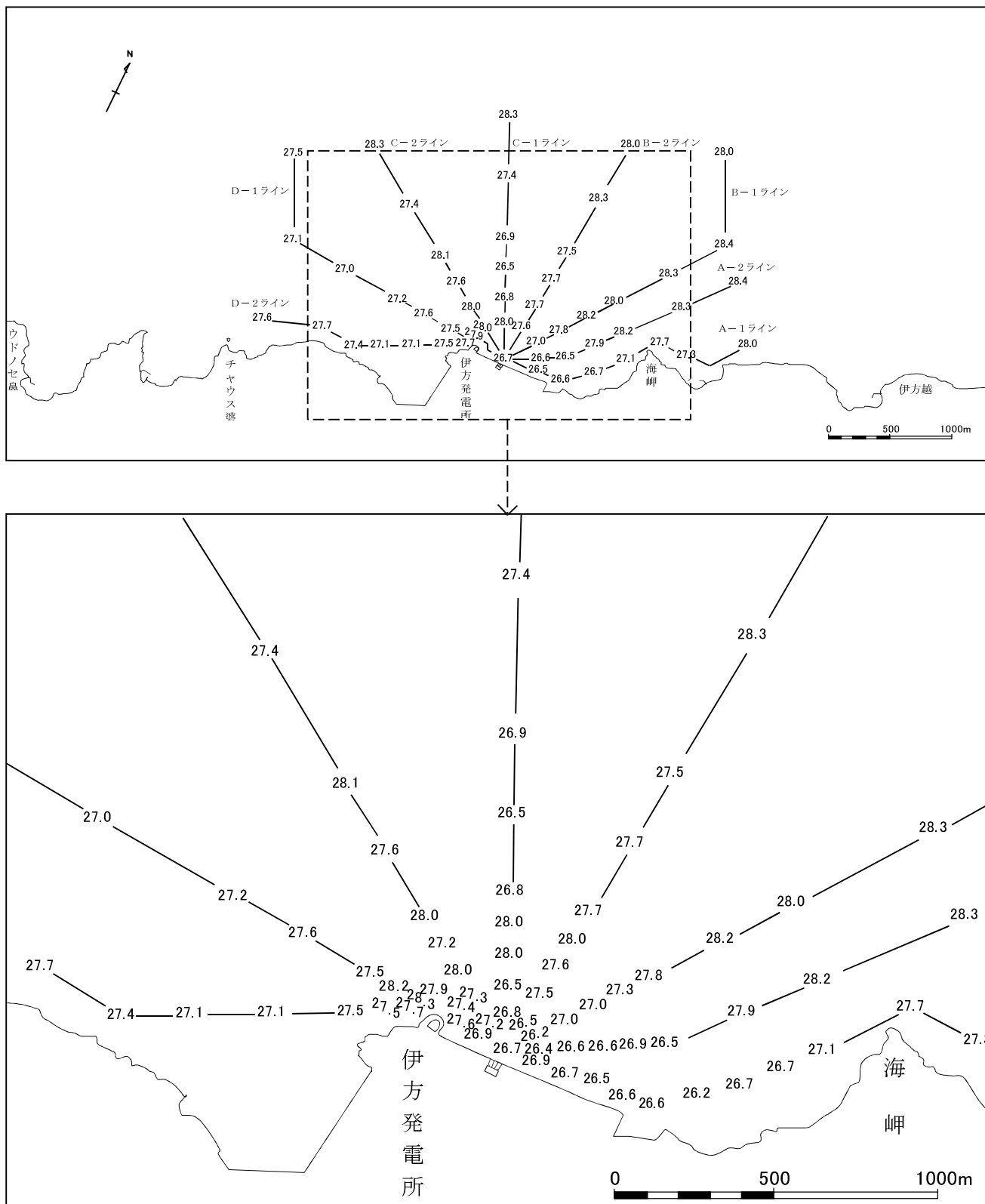
図 2 2 - ( 2 ) 水温水平分布調査結果 (夏季干潮時)
