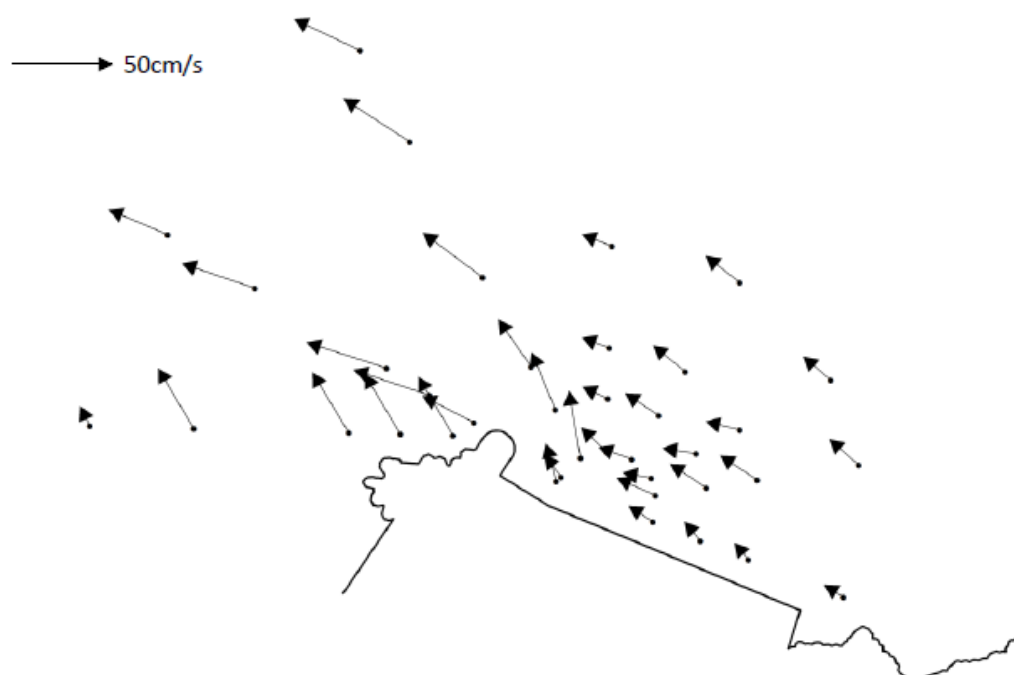
図20－（5）流動調査結果
