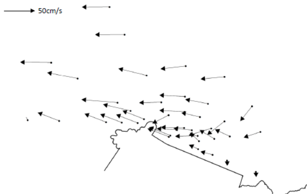
図20-（12）流動調査結果
