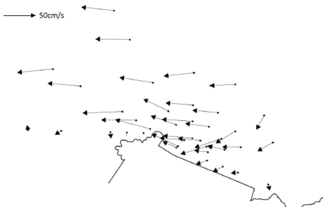
図20-（11）流動調査結果
