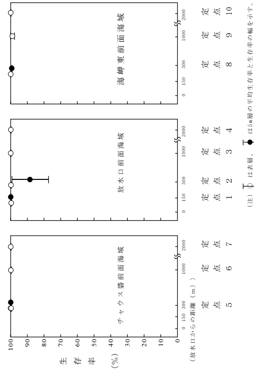
動物プランクトン(かいあい類)の生存率 (令和6年8月12日～13日)
