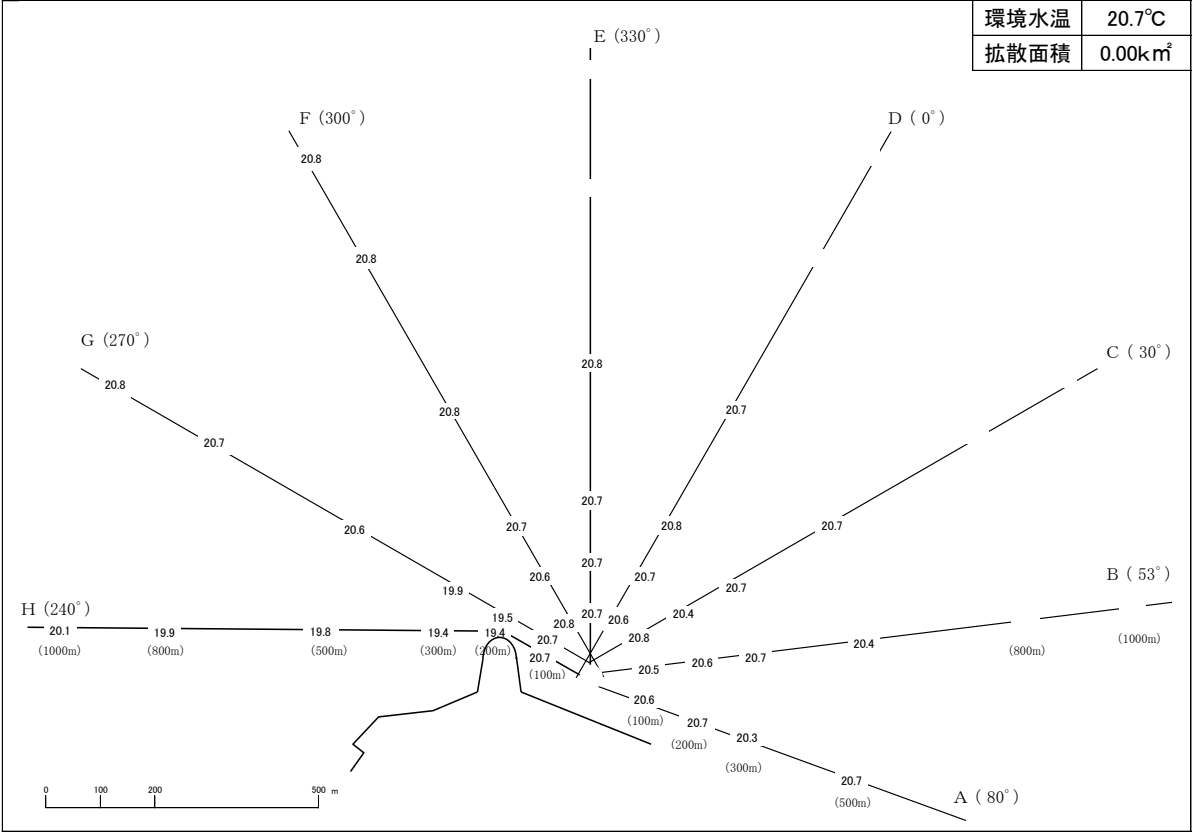
図 19－（5）温排水拡散状況調査結果
