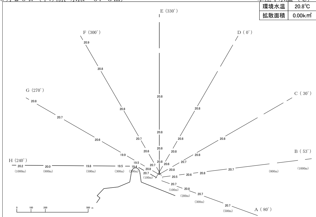
図 19 - （4）温排水拡散状況調査結果
