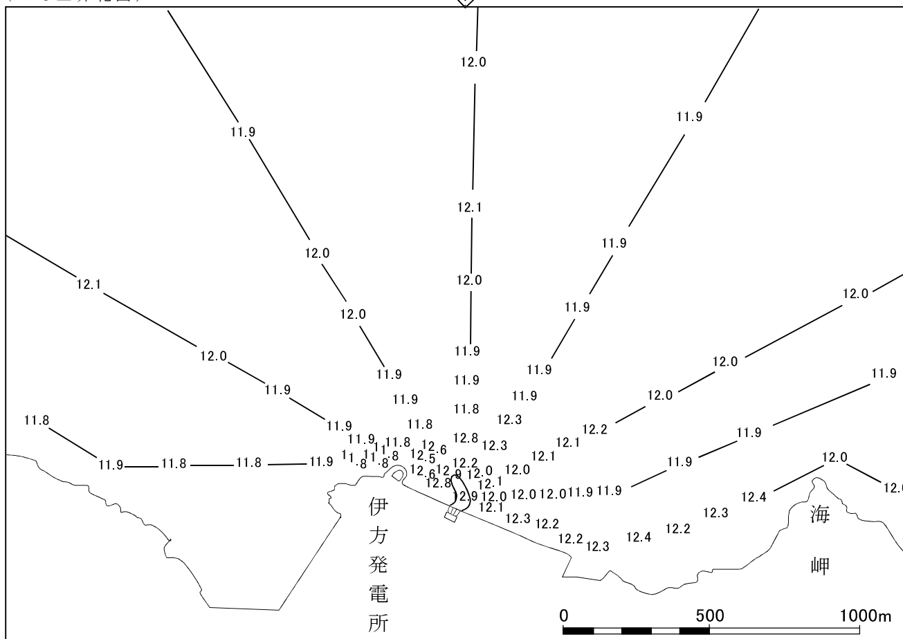
図 2 2 - ( 4 ) 水温水平分布調査結果 ( 冬季上げ潮時 )
