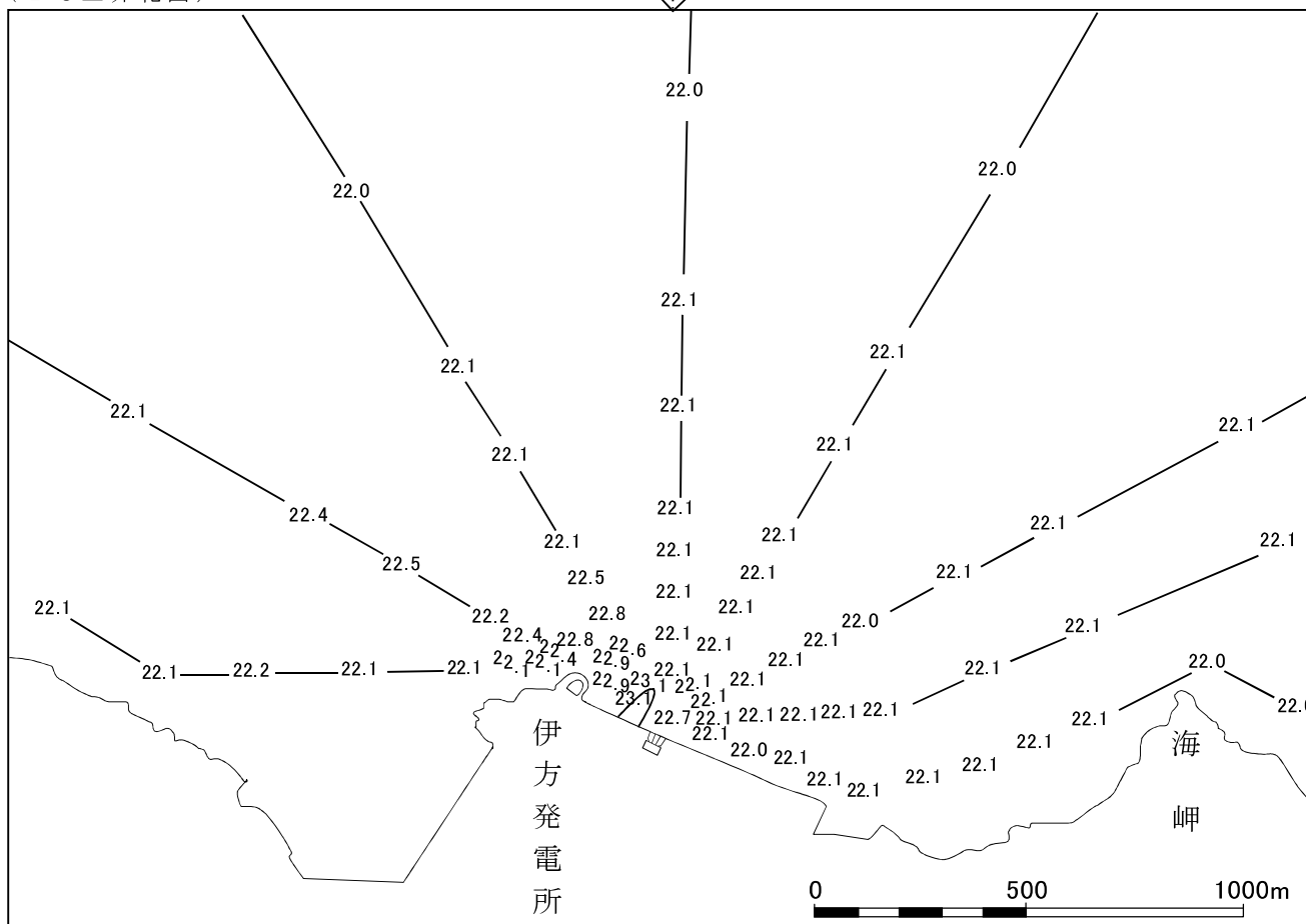
図 2 2 - ( 3 ) 水温水平分布調査結果 ( 秋季下げ潮時 )
