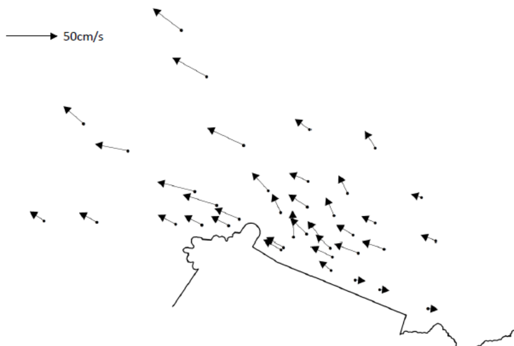
図20－（6）流動調査結果
