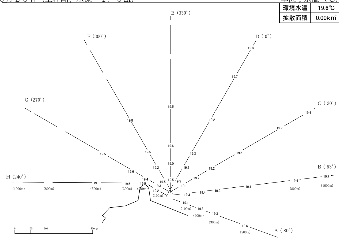
図19－（2）温排水拡散状況調査結果
