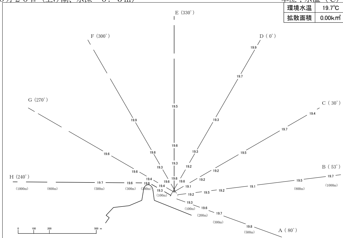
図19－（1）温排水拡散状況調査結果
