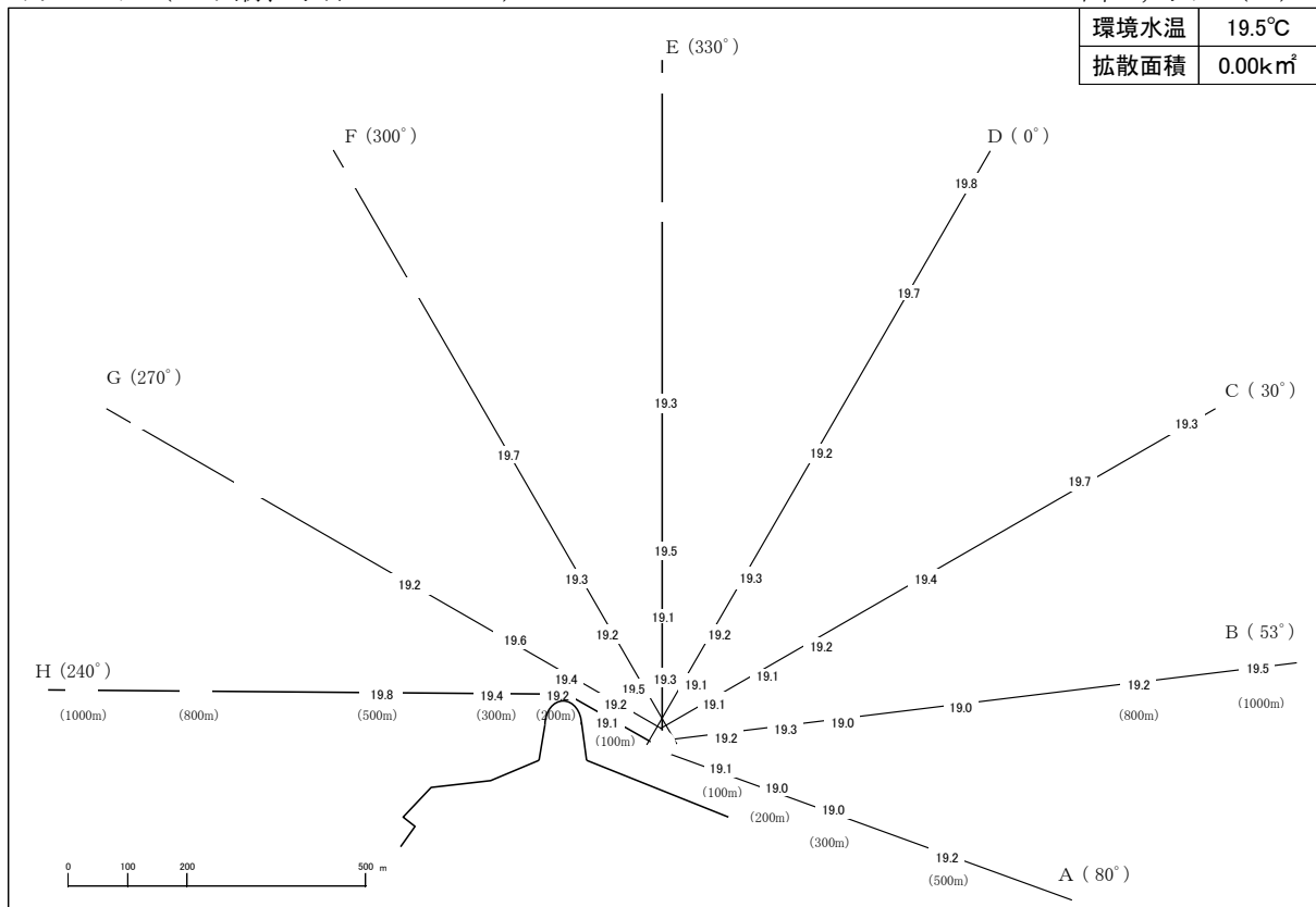
図 19 - （3）温排水拡散状況調査結果
