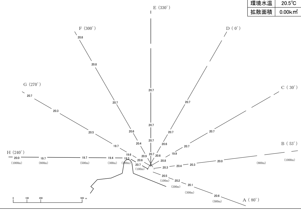
図 19－（6）温排水拡散状況調査結果
