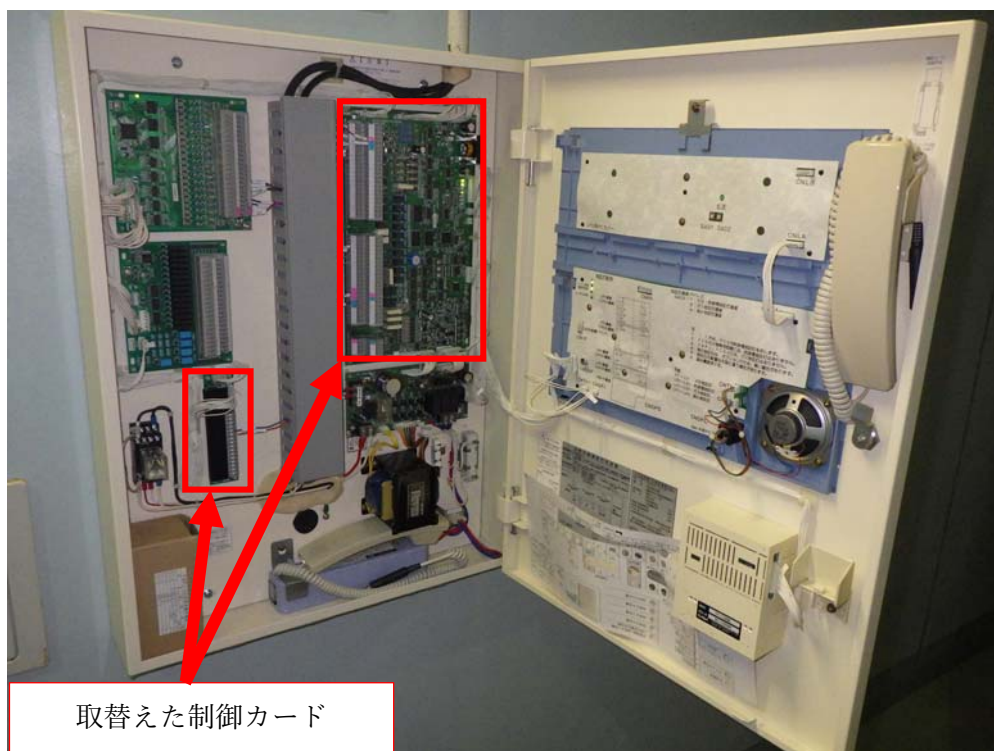
伊方3号機 純水装置建屋内 火災受信機盤 (復旧時)
