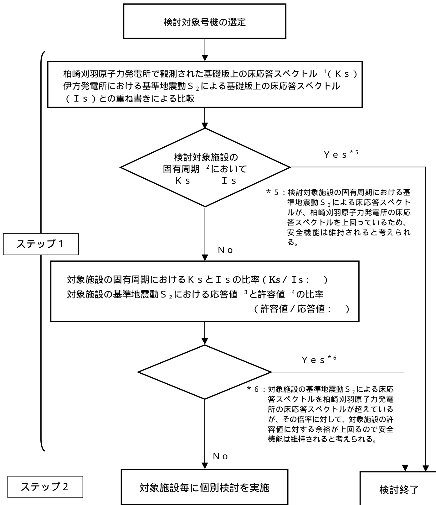
柏崎刈羽原子力発電所における観測データを基に行う 伊方発電所の主要施設への概略影響検討フロー図
