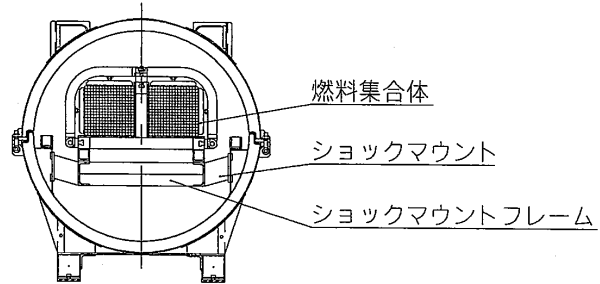
A-A断面
