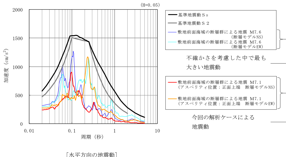
【図-2 今回の解析ケースの断層モデルによる地震動解析結果】
