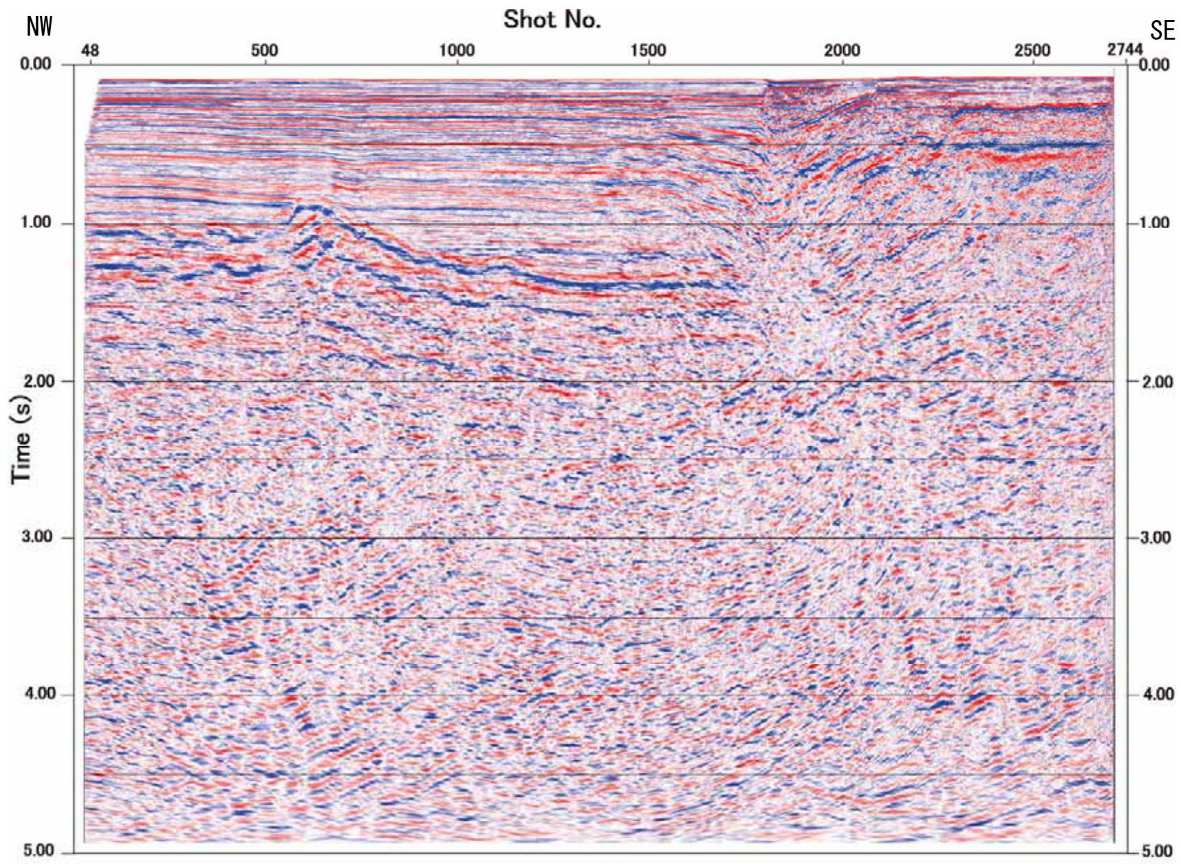
図-13 エアガンによる探査断面図（保内沖 時間断面）
