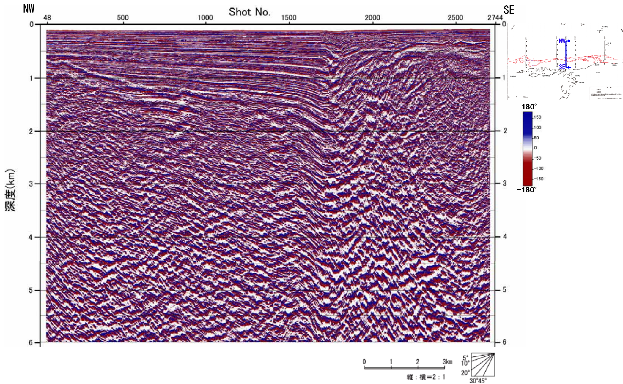
図-28 アトリビュート解析断面図 (伊方沖 瞬間位相)
