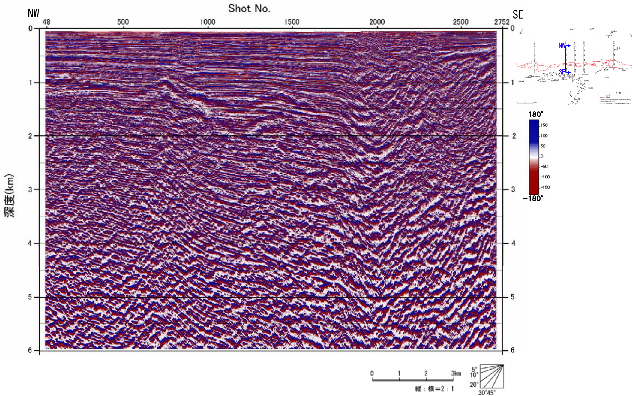
図-31 アトリビュート解析断面図（瀬戸沖 瞬間位相）
