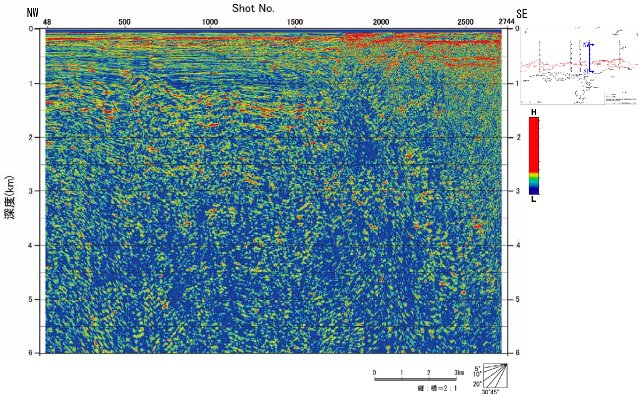
図-26 アトリビュート解析断面図 (保内沖 エンベロップ)
