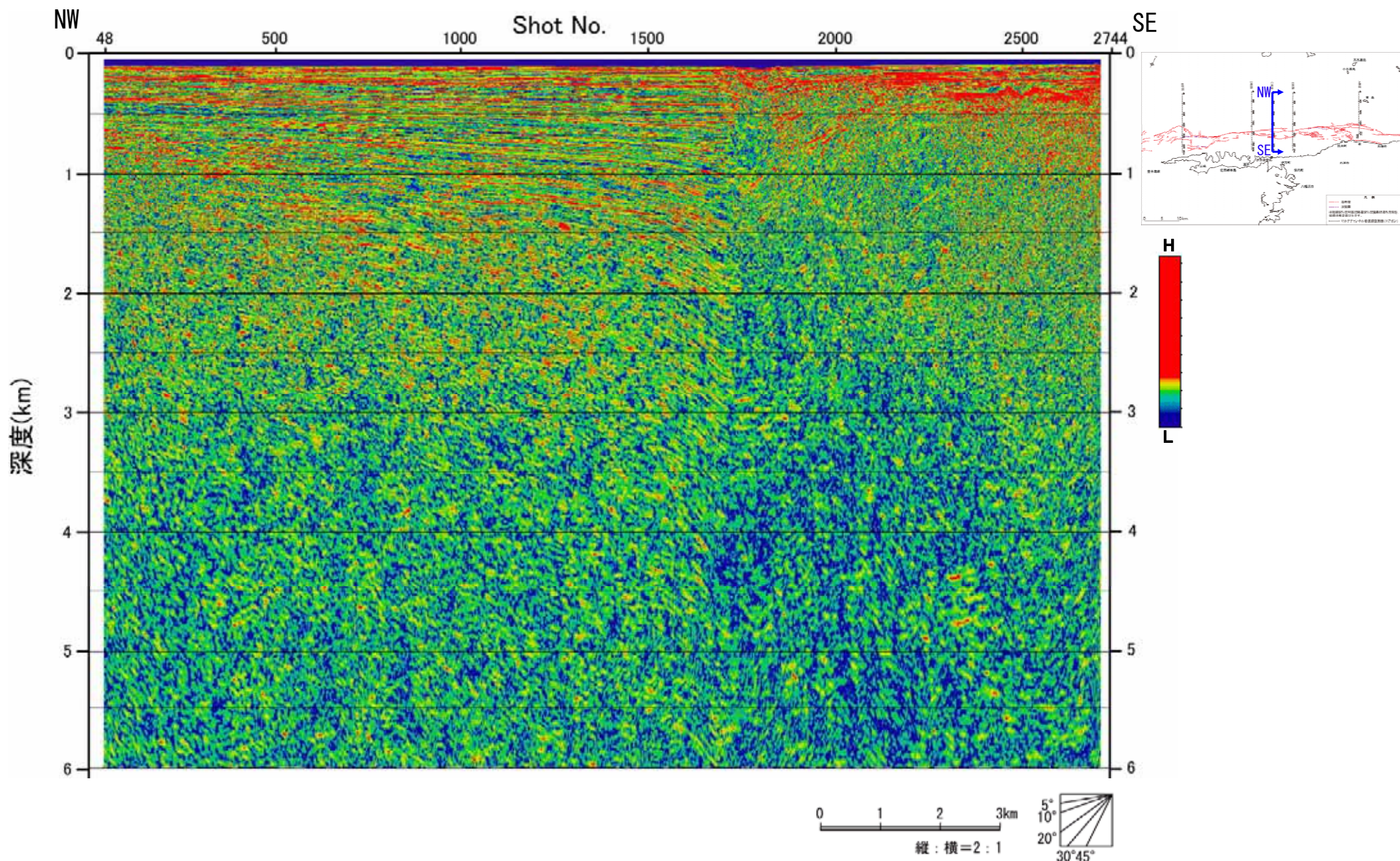
図-29 アトリビュート解析断面図（伊方沖 エンベロープ）
