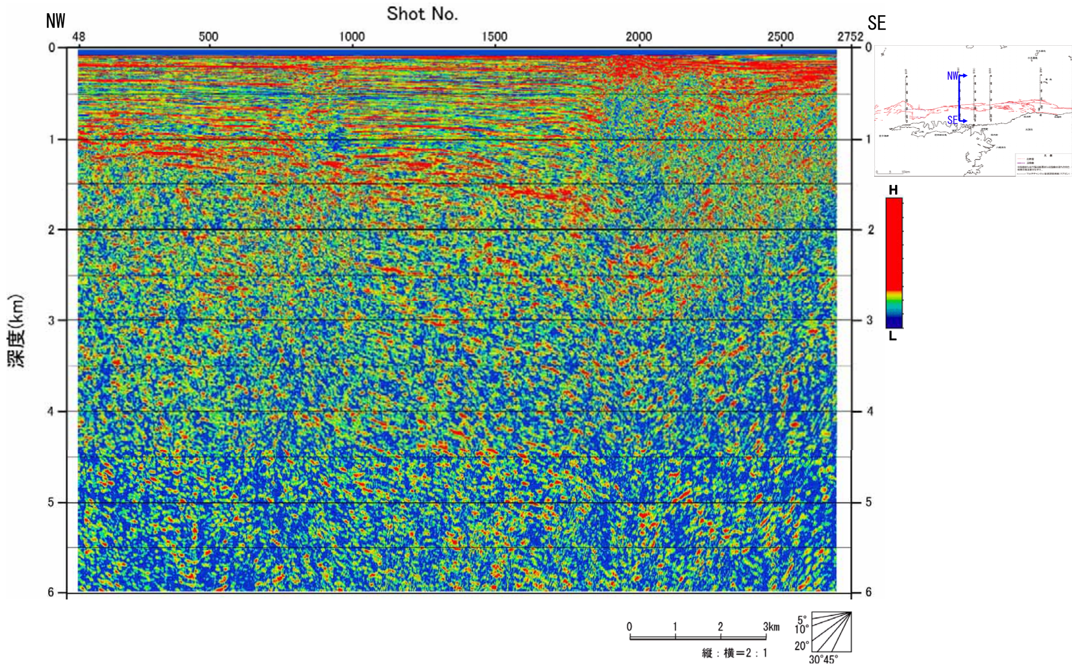
図-32 アトリビュート解析断面図 (瀬戸沖 エンベロープ)
