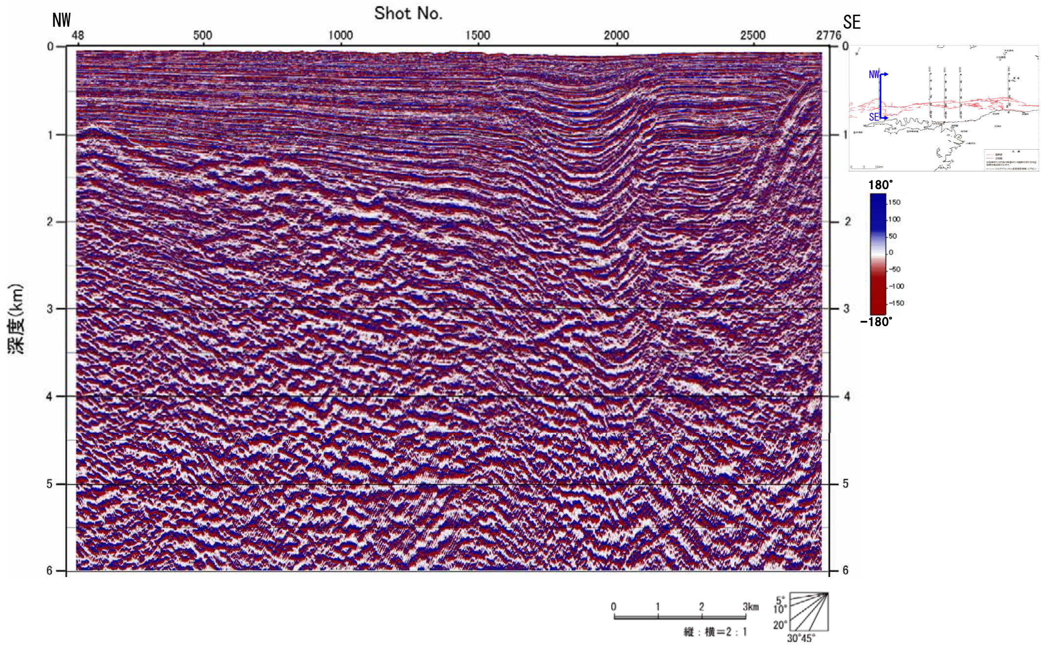
図-34 アトリビュート解析断面図（三崎沖 瞬間位相）
