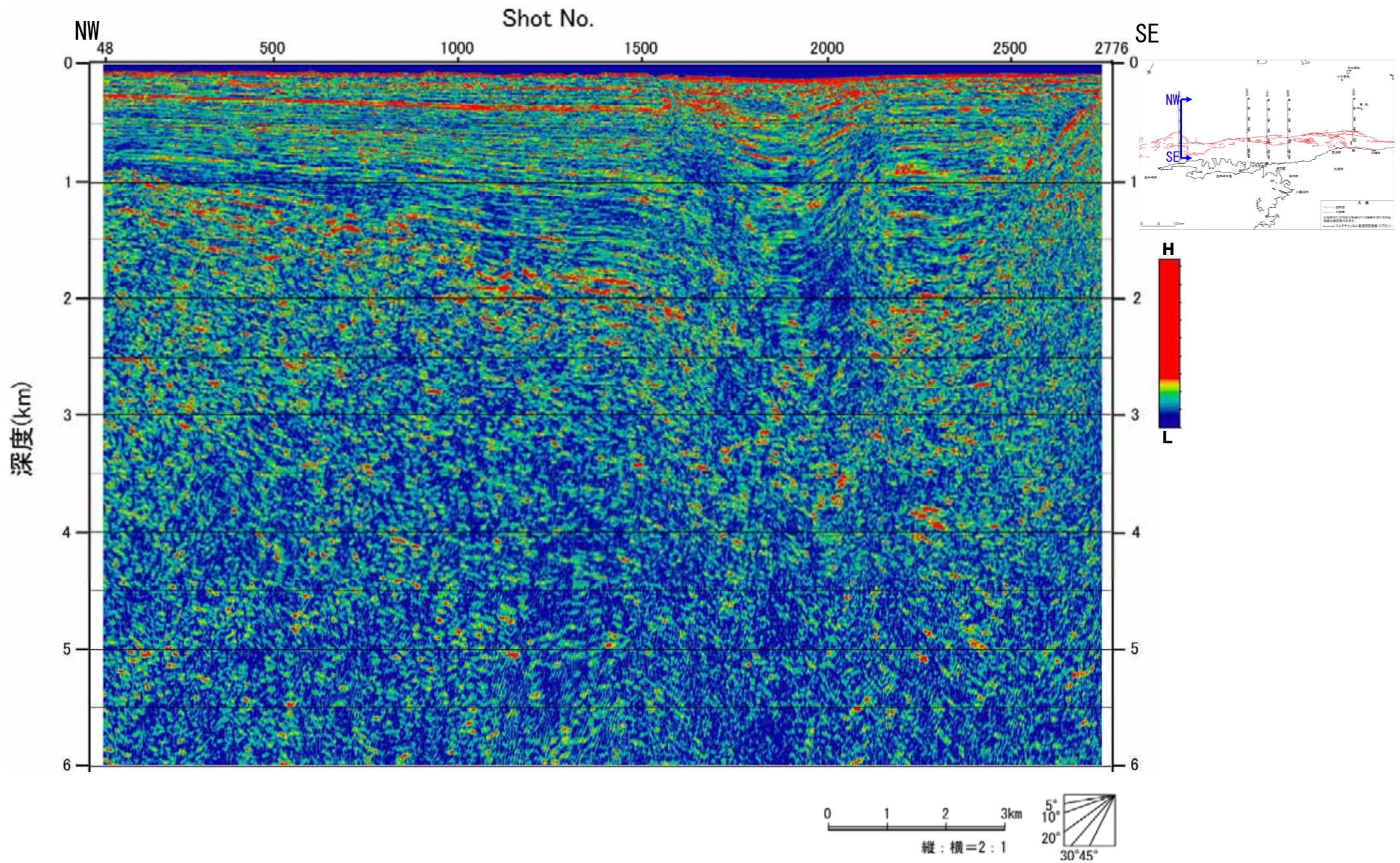
図-35 アトリビュート解析断面図 (三崎沖 エンベロップ)
