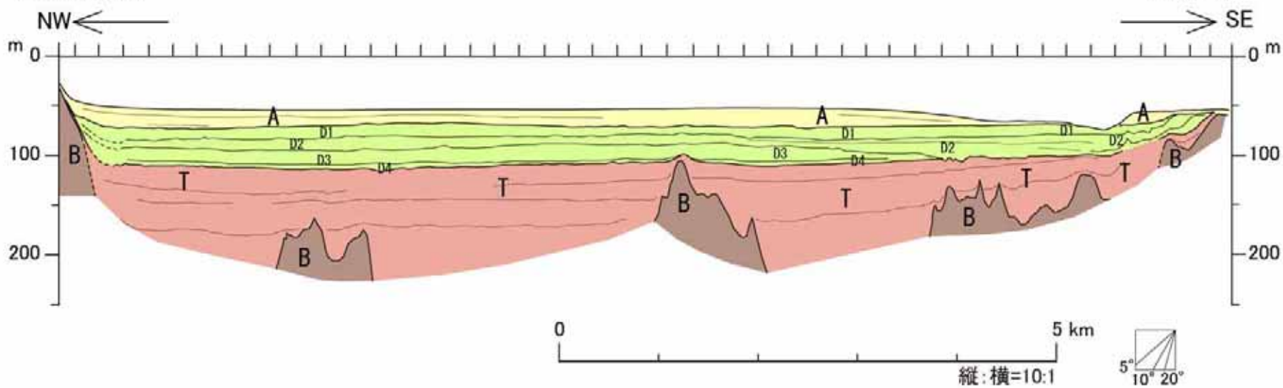
図-78 海底地質断面図(伊方発電所南方断面)
