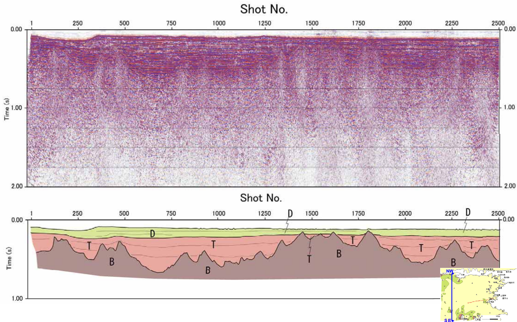
図-84 エアガンによる探査断面図（三崎南方断面）
