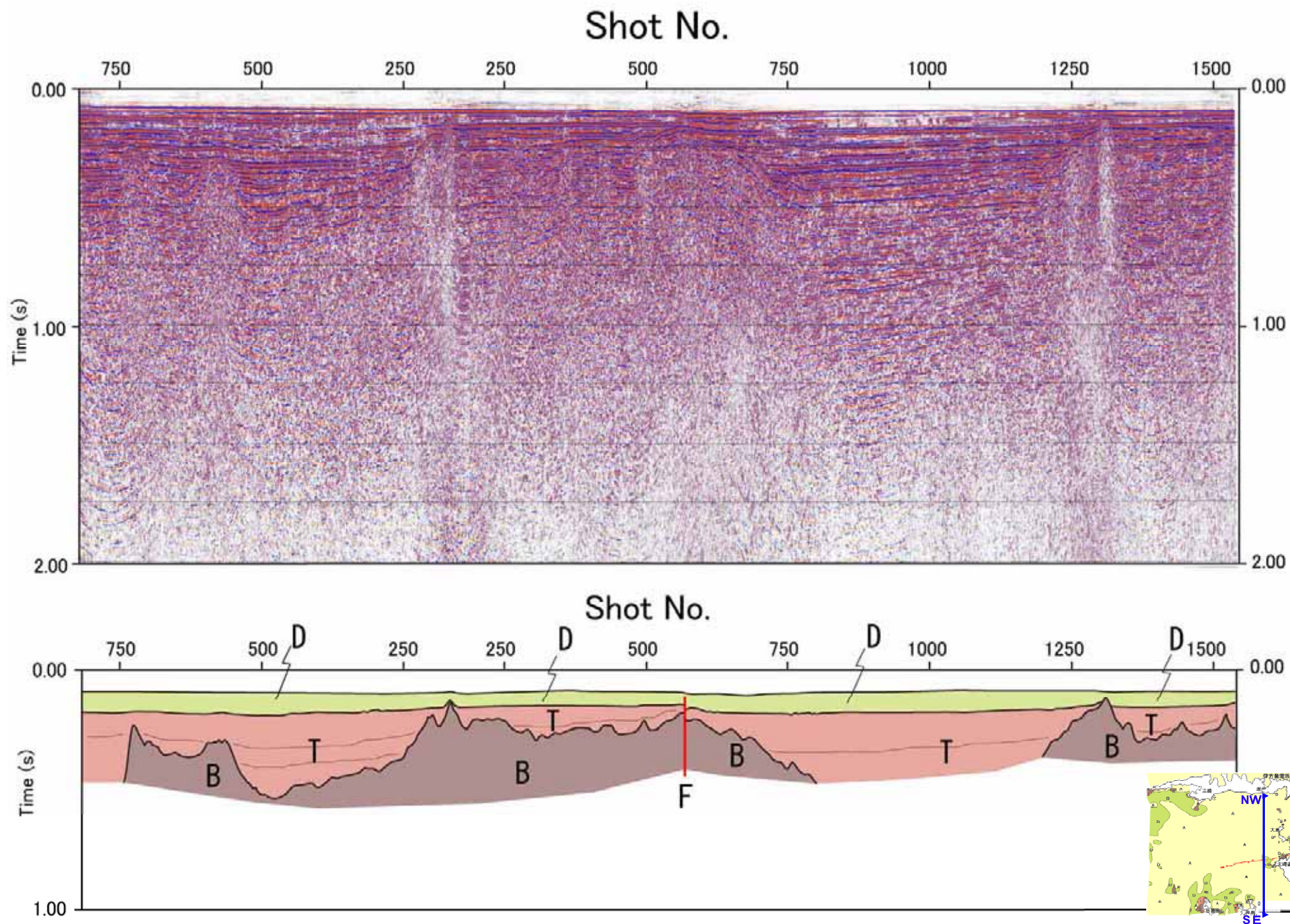
図-83 エアガンによる探査断面図（瀬戸南方断面）
