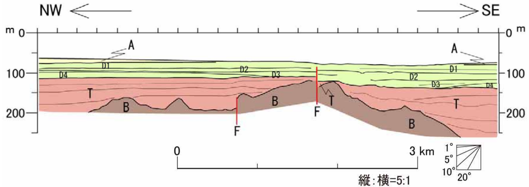
図-89 F-21 断層の海底地質断面図 (瀬戸南方断面)
