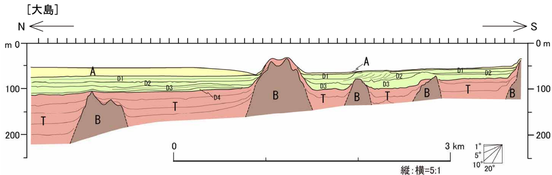
図-88 沿岸部の海底地質断面図 (大島東方断面)
