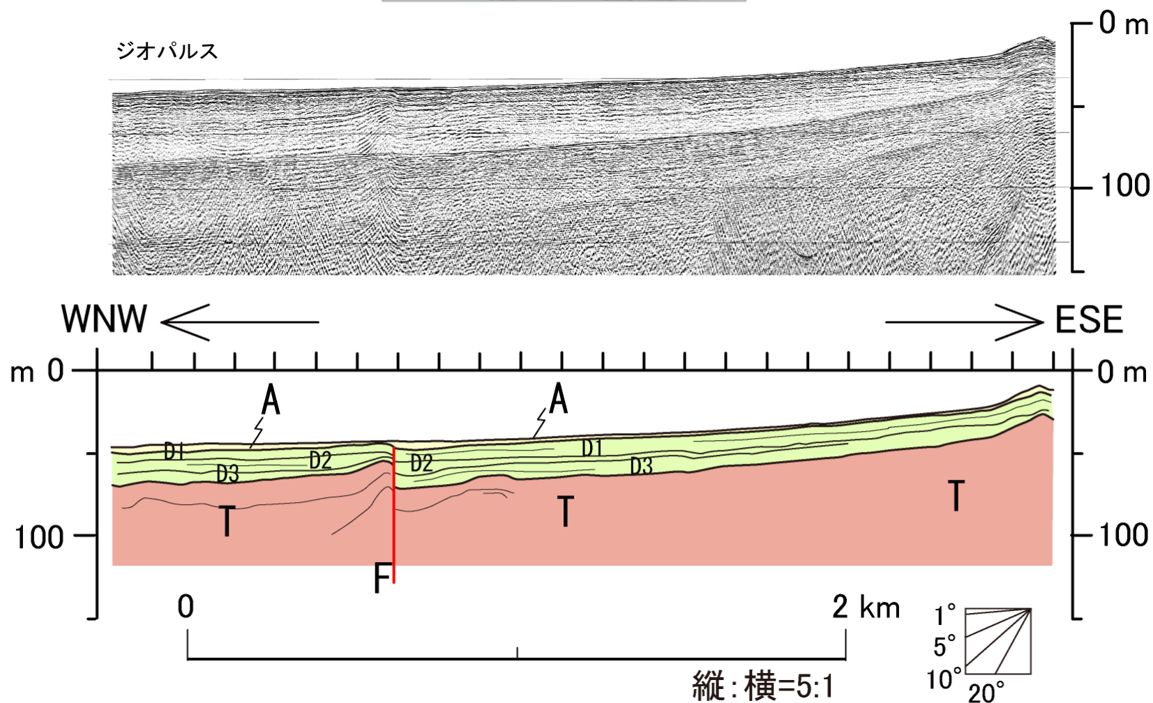
図-91 F-21 断層の海底地質断面図（東端付近）
