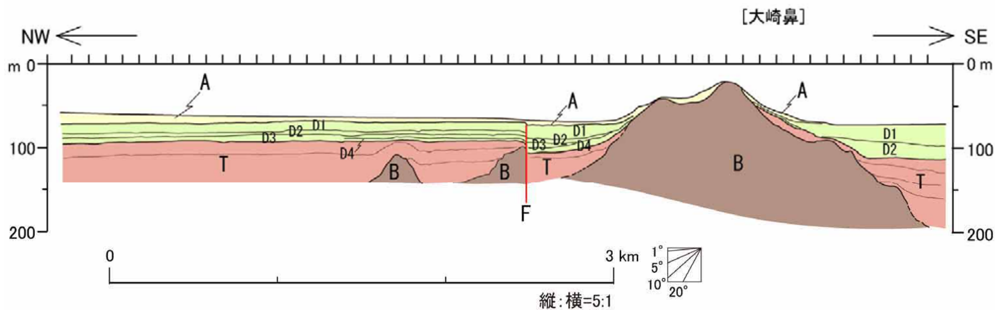
図-90 F-21 断層の海底地質断面図 (大崎鼻西方断面)
